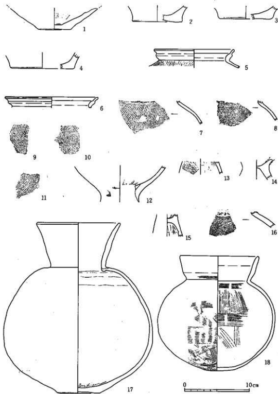
第2图 濛址15出土遗物
