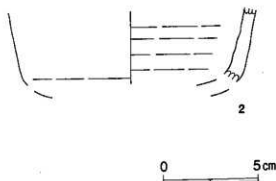
第9図 遺物実測図 (1/2)
