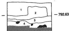
【No.2グリッド東面セクション図】
