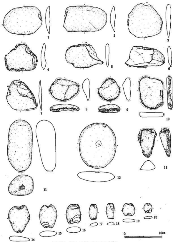
第218图 ARB 8号住居址出土石器(十)
