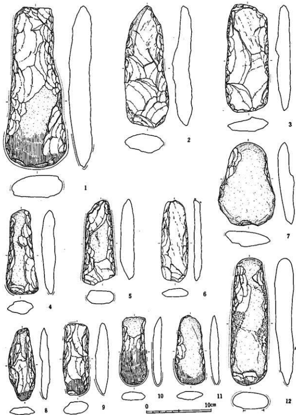
第138圖 GOB 遺構外出土石器(十)
