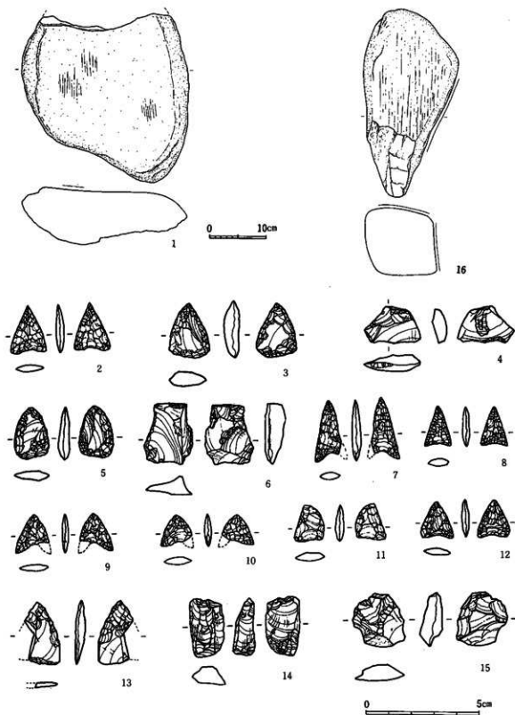
第166図 ARY 小竪穴5(1)、ユニット1(2-6)、ユニット2(7-11)、ユニット3(12-15)、 11号住居址(16)出土石器(号、1・16のみ寸)
