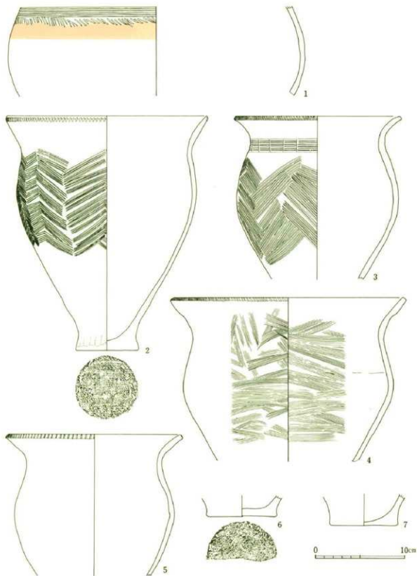
第156图 ARV 9号住居址出土土器(1/3)
