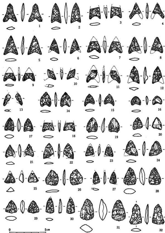
第181圖 ARV 遺構外出土石器(子)
