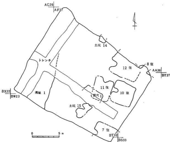
挿図4 遺構分布図
