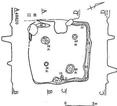
挿図7 10号住居址
