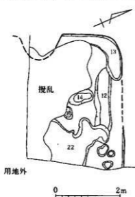
挿図5 7号住居址
