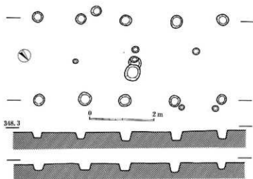
38図 ST103実測図 (1:80)
