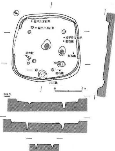
19 図 SA 106 実測図 (1 : 80)
