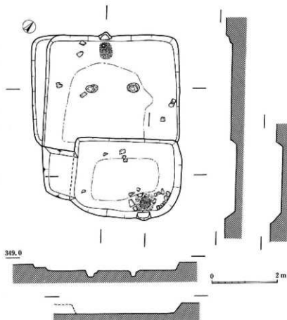
56図 SA6(下)・7(上)実測図(1:80)
