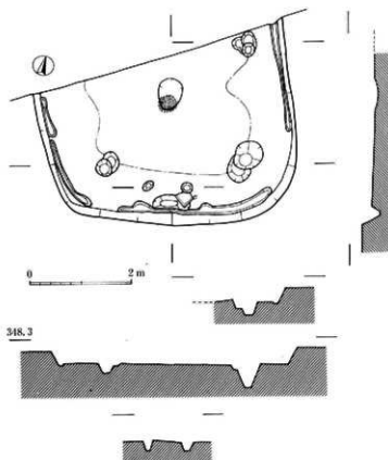
27図 SA109実測図 (1:80)
