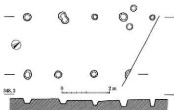
36図 ST101実測図 (1:80)
