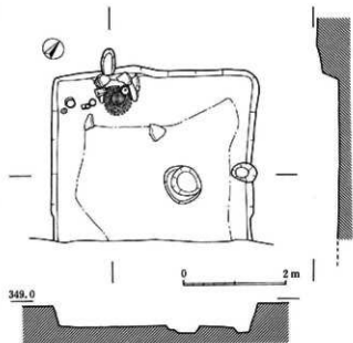
47図 SA1実測図(1:80)
