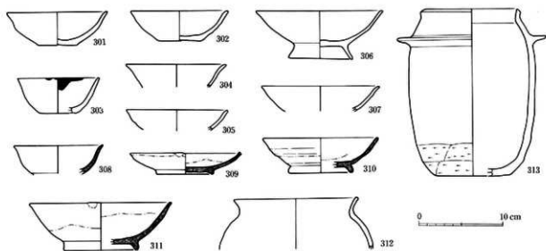
58 図 SA7 出土土器実測図 (1:4)
