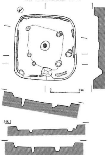
13図 SA103実測図(1:80)
