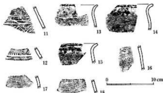
12図 SA102出土土器拓影(1:4)
