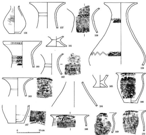
28 図 SA 109 出土土器実測図・拓影 (1:4)
