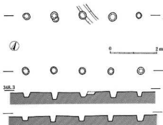
37図 ST102実測図 (1:80)
