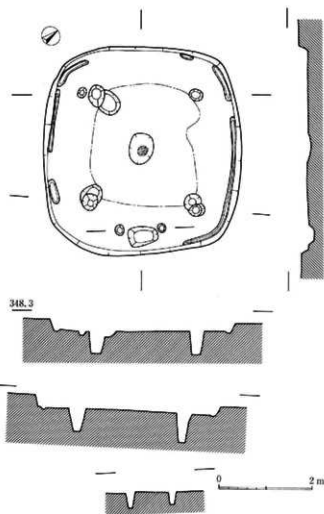
9図 SA101実測図(1:80)
