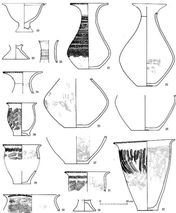
14図 SA 103 出土土器実測図 (1 : 4)
