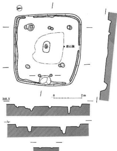
17図 SA105 実測図 (1:80)
