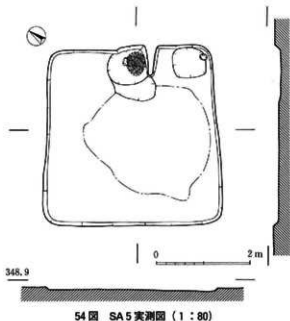
54 図 SA 5 実測図 (1 : 80)
