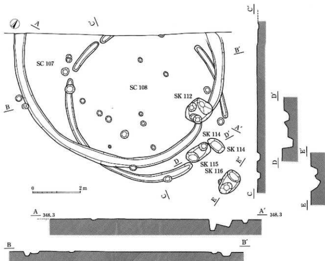
35図 SC 107・108、SK 112・114～116実測図 (1:80)
