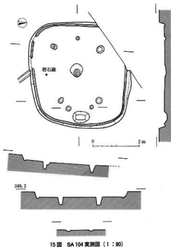
15図 SA104実測図(1:80)
