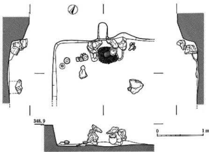
48図 SA1カマド実測図(1:40)
