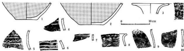
10図 SA101出土土器実測図・拓影(1:4)
