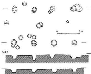
40図 ST107実測図(1:80)
