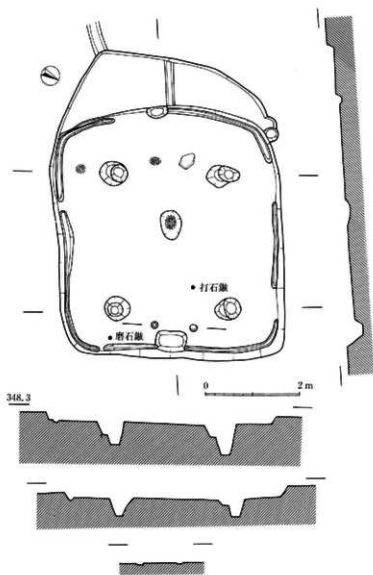
25図 SA 108 実測図 (1:80)
