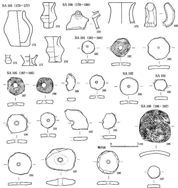
43 図 土製品・ミニチュア土器実測図 (1 : 2)
