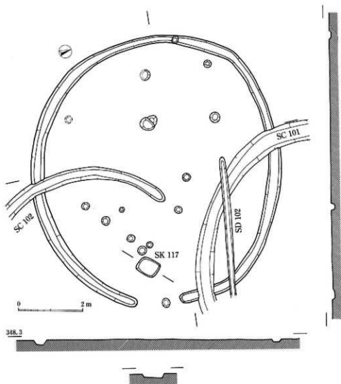
31 図 SC103、SK117 実測図 (1:80)
