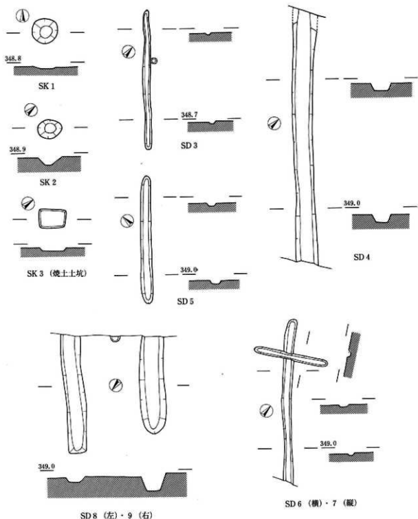
59 図 土坑・溝址実測図 (1:80)
