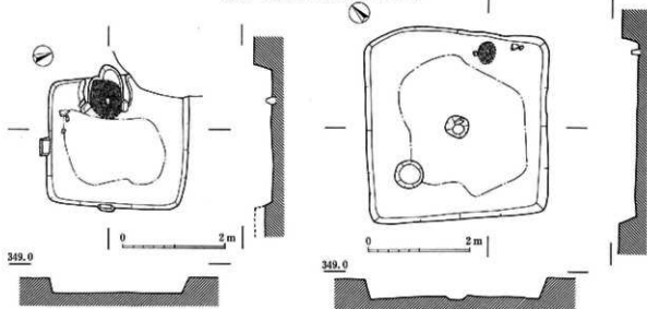
51図 SA2実測図(1:80)
