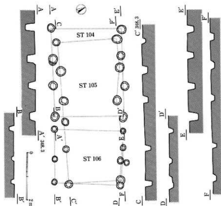
39図 ST104~106実測図(1:80)
