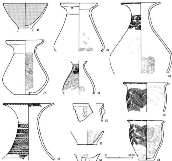
18図 SA105 出土土器実測図 (1:4)
