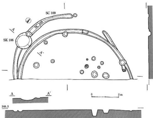
34 図 SC106・109、SK106実測図 (1:80)
