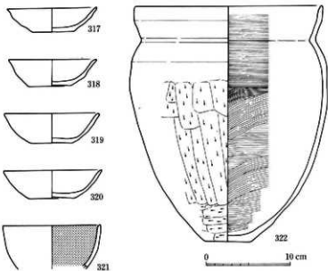
61 図 検出出土土器実測図(1:4)
