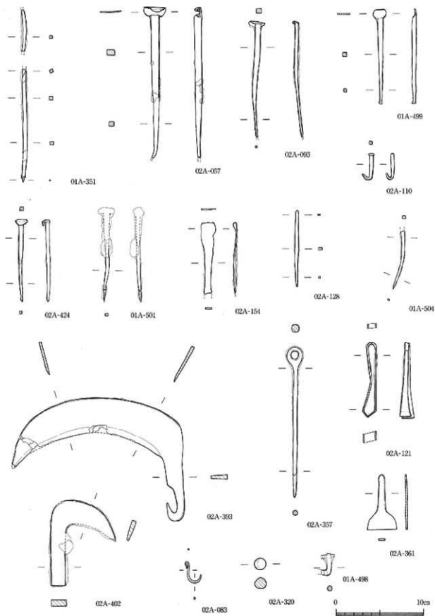
第84图 鉄製品実測図② (S=1/3)
