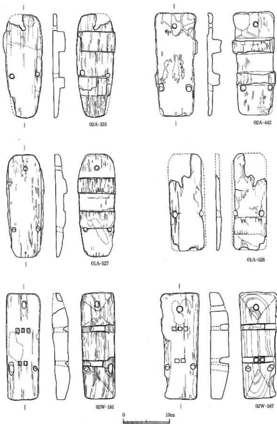
第96图 木製品実測图① (S=1/4)
