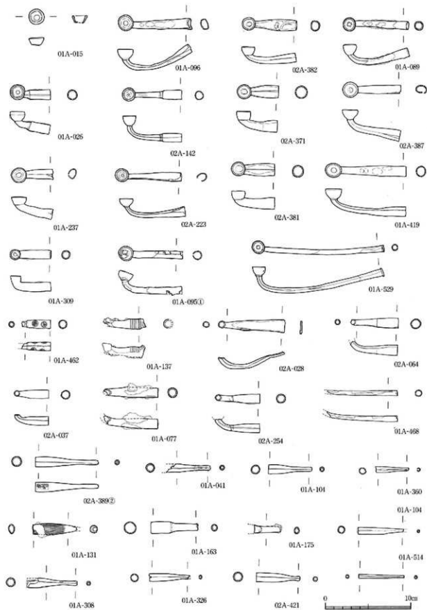
第91图 烟管类测图① (S=1/3)
