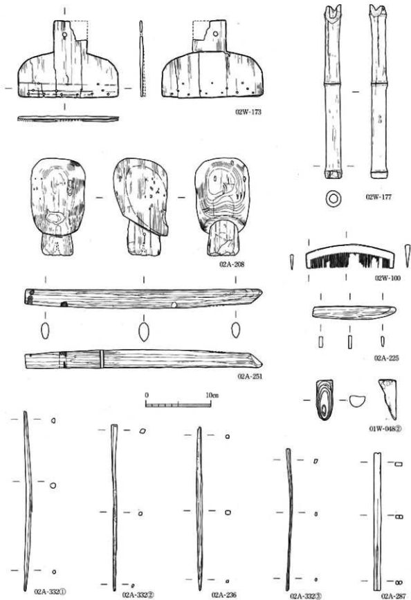
第97图 木製品実測図⑤ (S=1/4)
