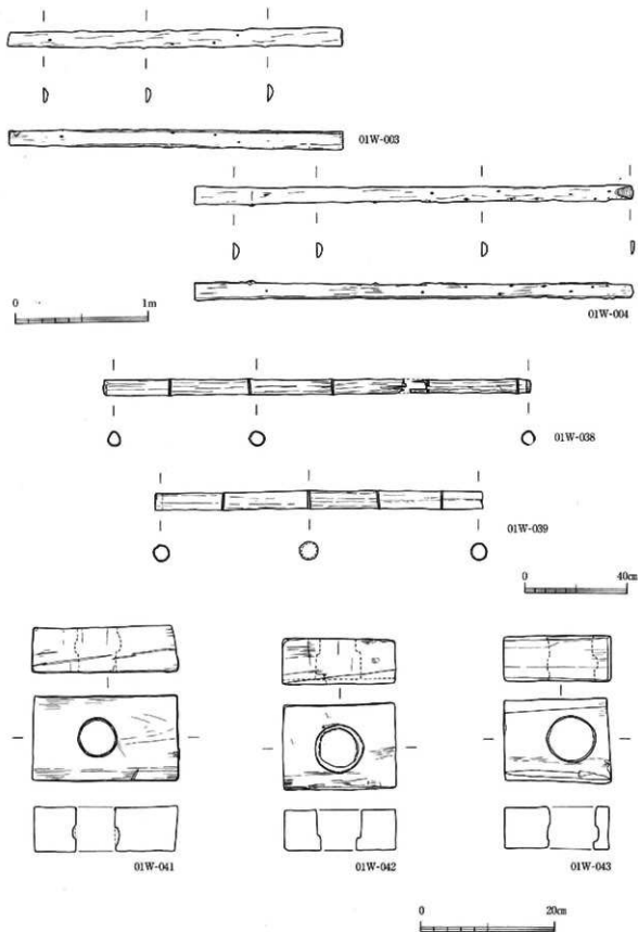
第100图 木製品実測図⑧ (S=1/6, 1/16, 1/30)
