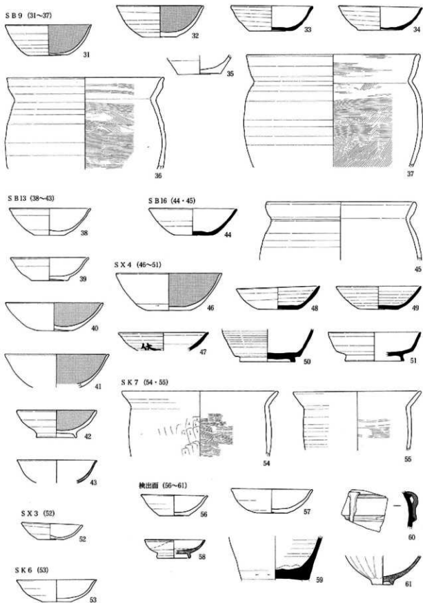
13图 SB 9・13・16、SX 3・4、SK 6・7 検出面出土土器実測図 (1:4)
