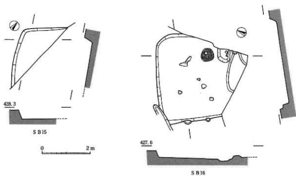
10图 SB 4 · 5 · 8 · 15 · 16, SK 2 · 5 实测图 (1:80)
