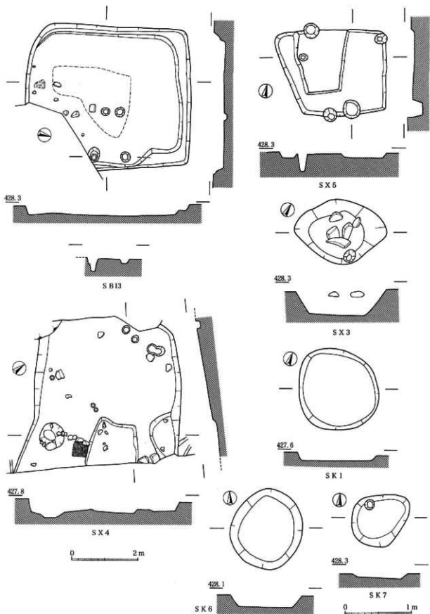
11図 SB13、SX3～5、SK1・6・7実測図 (1:80、SX3およびSK1は1:40)
