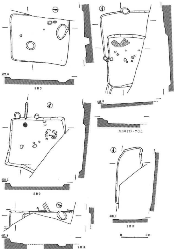
9图 SB 3 · 6 · 7 · 9 · 12 · 14実測图 (1:80)
