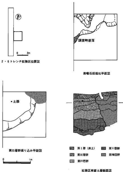
第33図 2・6トレンチ拡張区黒曜石採掘坑実測図 (1/40)
