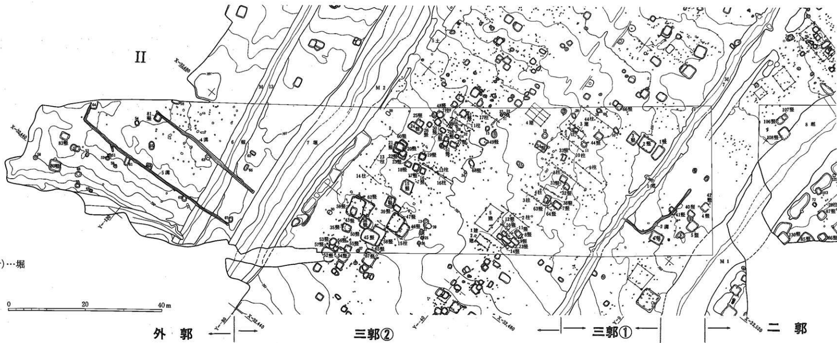
付図1 金井城跡遺構配置図 (1:500)
