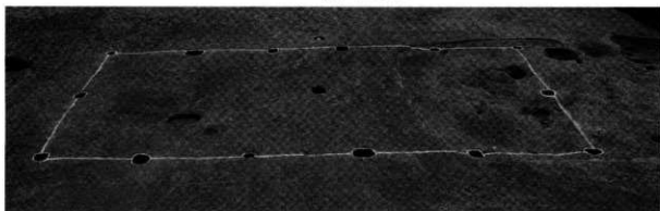
III-16 2号掘立柱建物址
