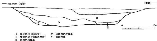
第27図 1号溝断面図
