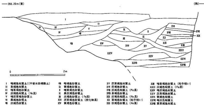
第12图 10号溝断面图
