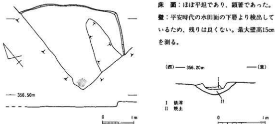
第5図 1号住居跡及び炉断面
