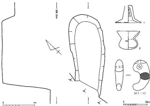
第11图 9号土坑及出土遗物
