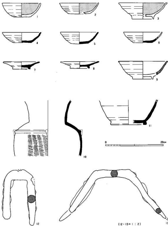
第20图 16号住居跡出土遺物
