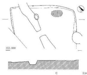
図31 SB23実測図 (S = 1 : 80)
