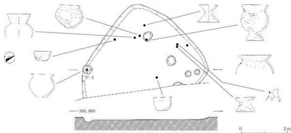
図36 SK95実測図（S=1:80）（土器、S=1:8）
