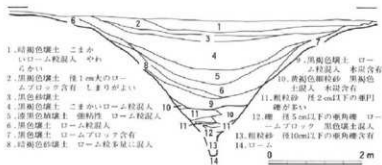
第19図 上木戸遺跡101号溝断面図(1:80)
