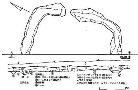
第15図 犬原遺跡1号方形周溝墓(1:80)
