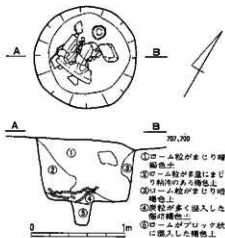
第14図 犬原遺跡3号土塚(1:40)
