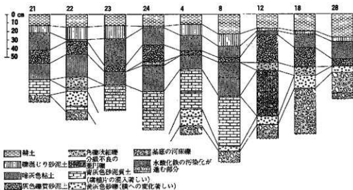
第40回 高田遺跡柱状断面図No.4
