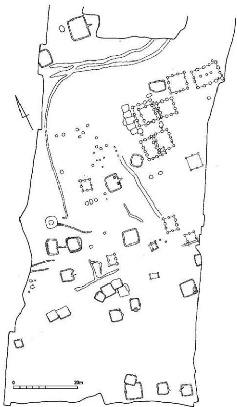
第38図 三の宮遺跡南端部遺構全体区(1:600)
