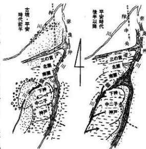
第5図 地形形成過程
