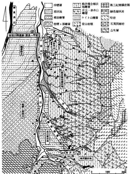
第2区 堀川市東部の地質図 (▲ 縄文時代中期を主体とする遺跡、○ 嶺高地)
