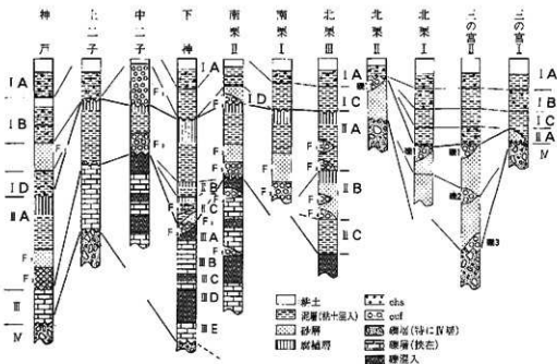
第3図 各地区基本層序
