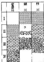
第4図 各河川の堆積傾向
