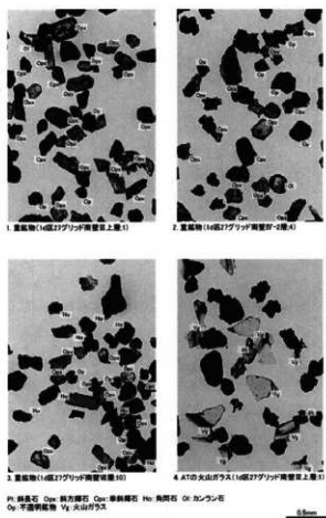
図13 重鉱物・火山ガラス顕微鏡写真
