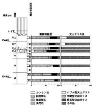
図14 16区27グリッド南壁深掘地点の重鉱物組成および火山ガラス比
