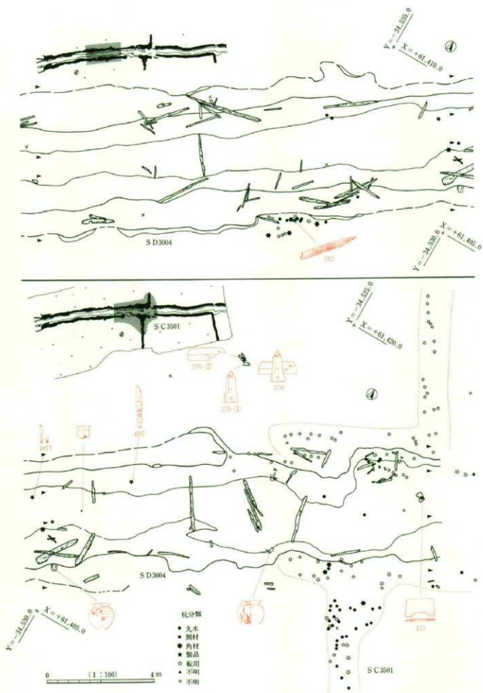
第154图 SD3004II、SC3501 平面·出土主要遺物分布图
