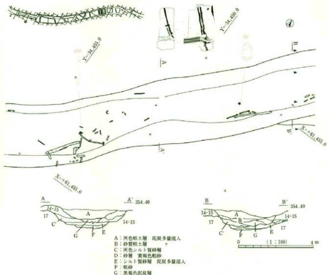
第177図 SD3004 (⑪-Ⅰ区古墳前期-) 平面・断面・出土主要遺物分布図
