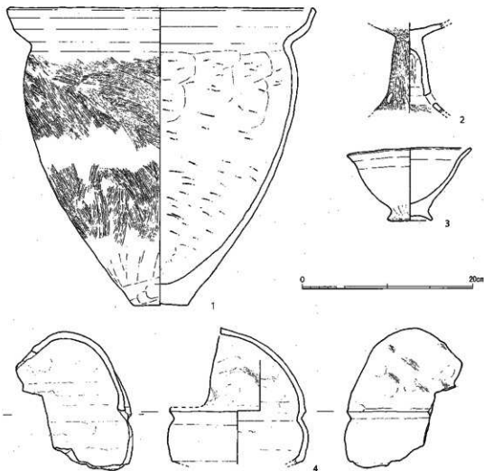
第6図 第2調査区出土遺物実測図
