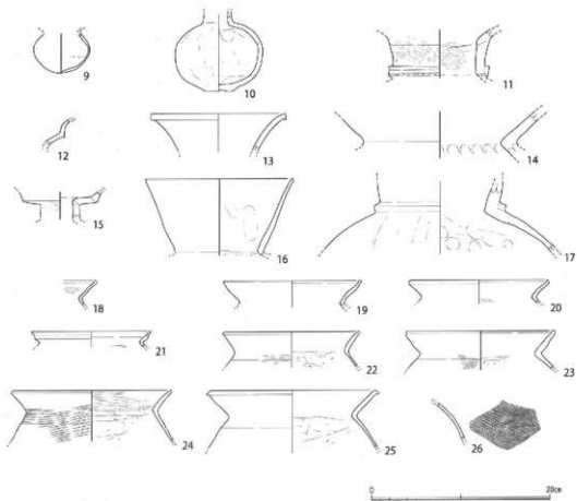
第10圖 出土遺物実測図(1)
