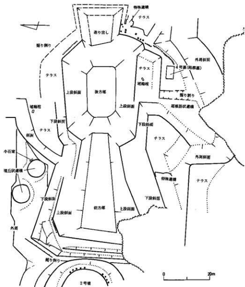
図7. 赤土山古墳の墳形推定図 (S 1/800)
