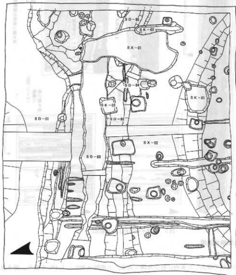
図4 遺構平面図および土層図1
