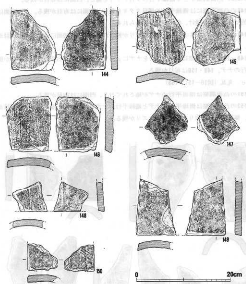
図15 出土瓦類実測図3 (S=1/4)
