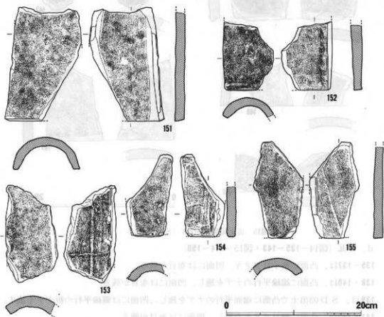
図16 出土瓦類実測図4 (S=1/4)
