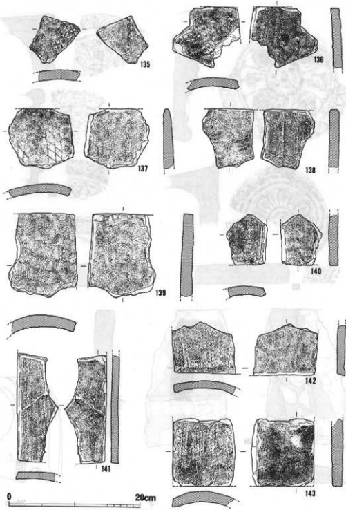
图14 出土瓦类实例图 2
