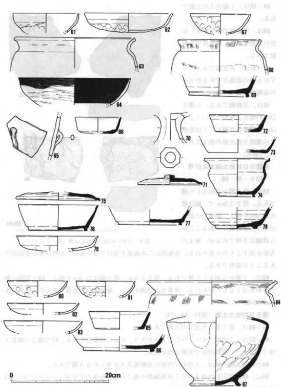
图10 SD-02·SD-03出土土器实测图(S=1/4)
