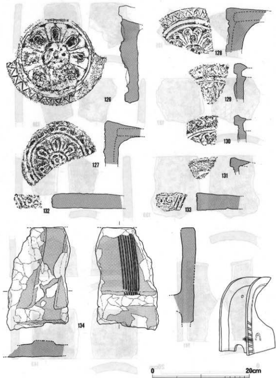
图13 出土瓦類実測図1 (S = 1 / 4)
