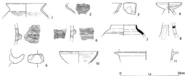
第5図 出土遺物実測図
