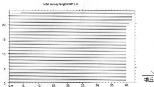
第14図 地中レーダ探査の測線 (縦軸がX、横軸がY)
