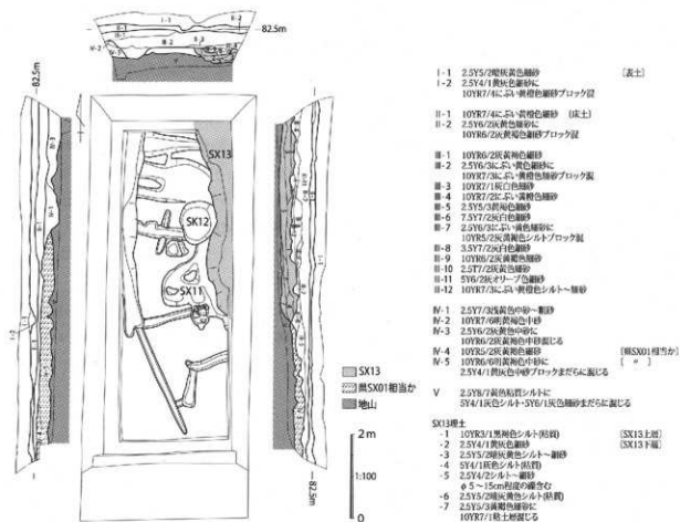
第4図 調査区平面図・土層図
