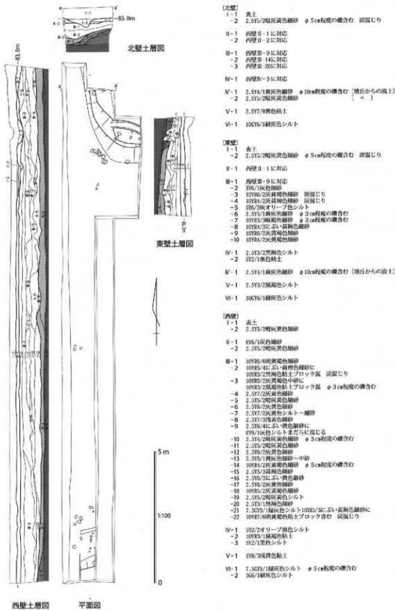
第9図 第1調査区平面図・土層図
