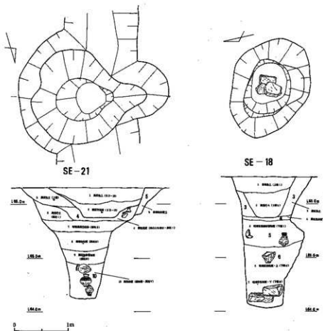
図5 弥生時代の井戸遺構図 (S1/50)
