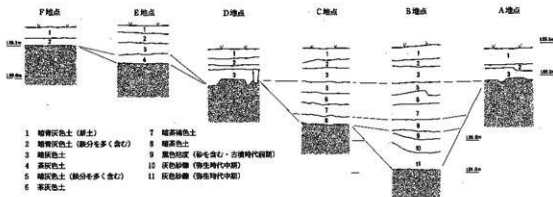
図3 基本土層図 (S 1/60)
