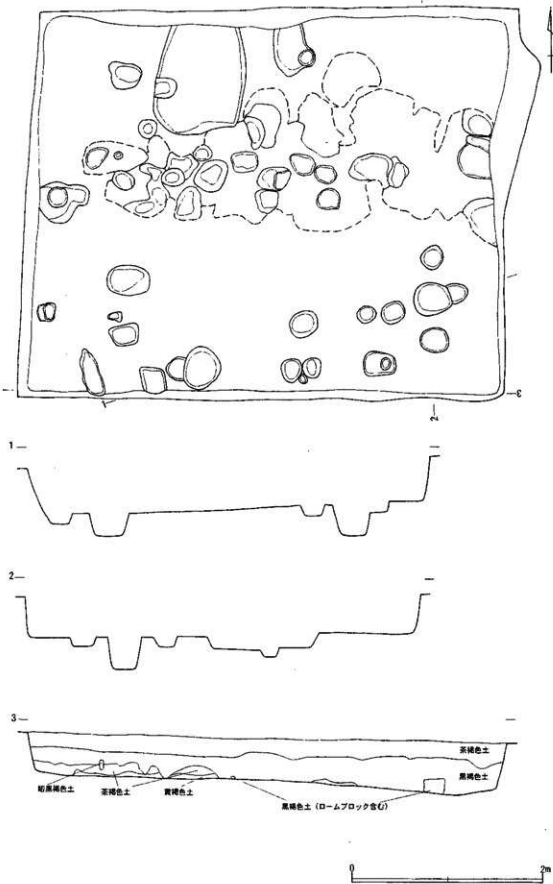
図4 調査区遺構分布図 (1:40)
