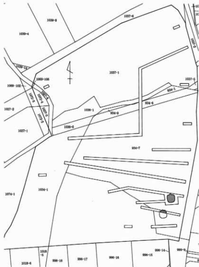
試掘調査全体図 (1:1,000)
