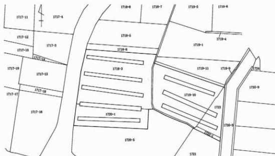
試掘調査全体図（1：1,000）
