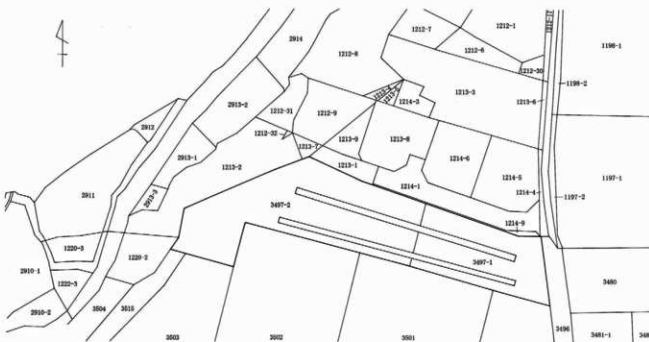
試掘調査全体図 (1:1,000)
