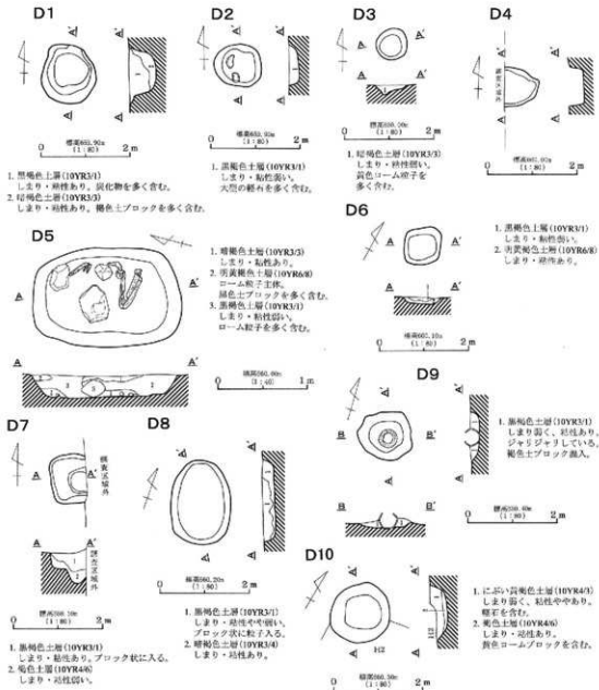
第12図 土坑実測図
