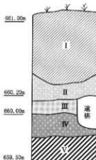
第2図 標準土層模式図
