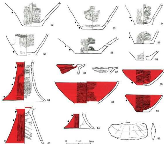
第41図 M7号溝状遺構出土遺物実測図②
