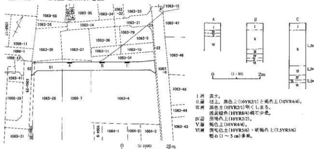
第25図 調査地点東地区全体図
