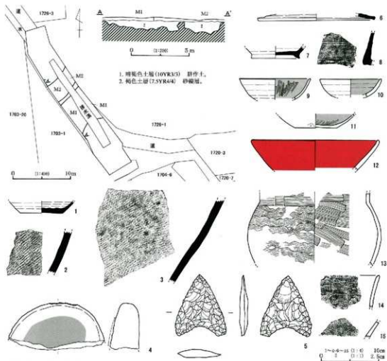
第46図 溝状遺構及び出土遺物実測図
