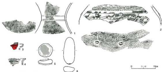
第9図 H4号住居址出土遺物実測図
