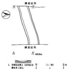
第7図 1号溝状遺構実測図
