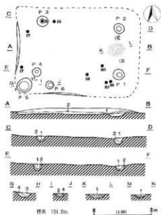
第8図 H5号住居址
