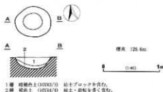
第20図 D 2号土坑
