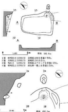
第34図 H1号住居址
