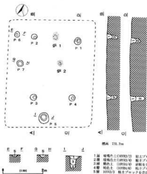
第12図 H7号住居址
