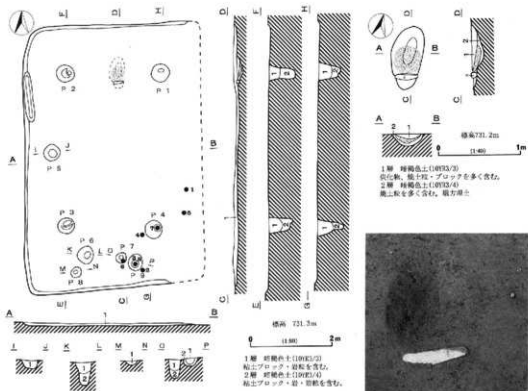
第10図 H 6号住居址
