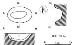
第22図 D 4号土坑
