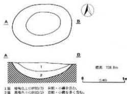
第21図 D 3号土坑
