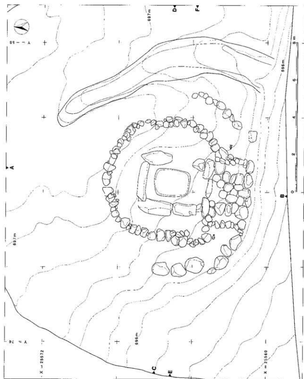
第25図 東久保古墳群1号墳の礎石と基礎地形(1:100)
