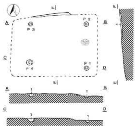
第17図 H11号住居址
