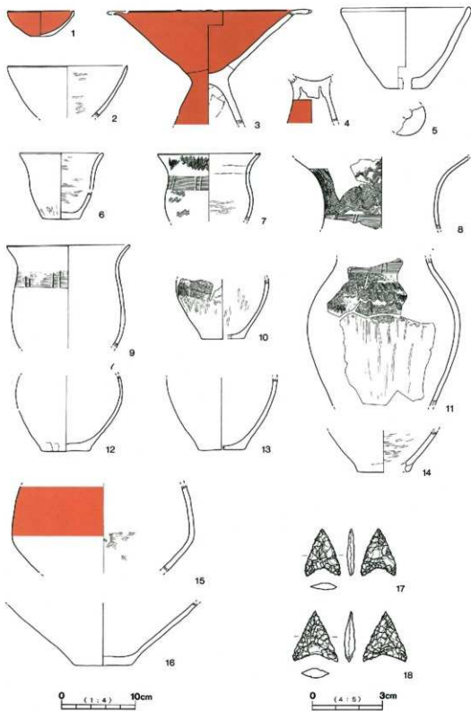
第7図 H4号住居址の土器と石器
