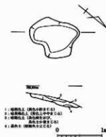
第5図 不明遺構実測図
