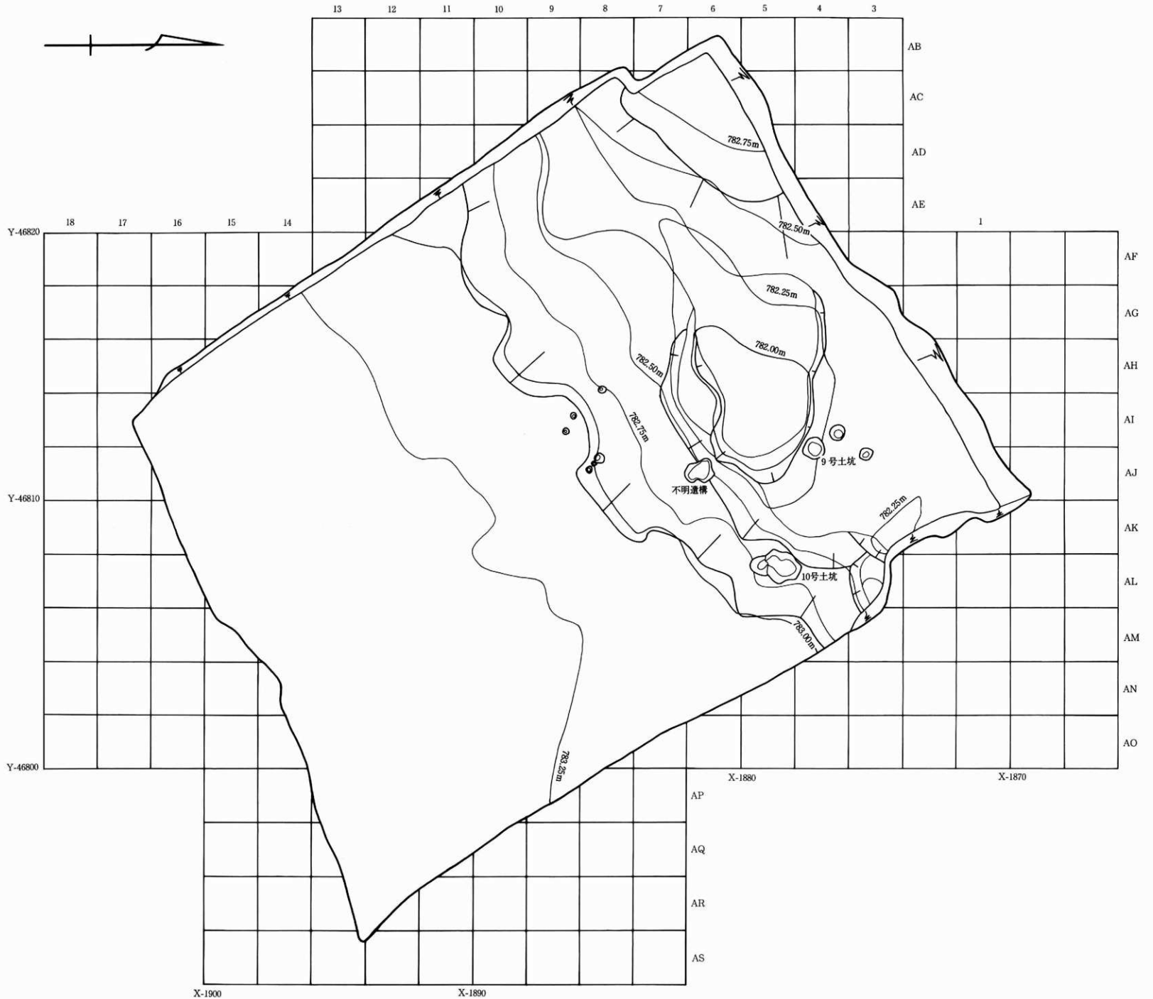
付图1 北潞舟A遺跡第1調査区全体測量図 (S = 1/100)
