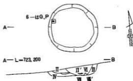
第11図 第1号土壌実測図(S=1/60)
