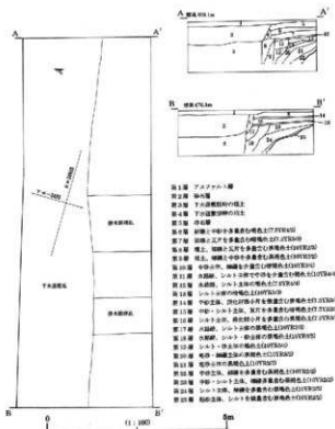
第21図 調査第⑥東区全体図 (1:100)
