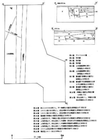
第23図 調査第②西区全体図 (1:100)
