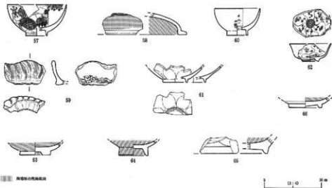
第26图 出土遺物実測図
