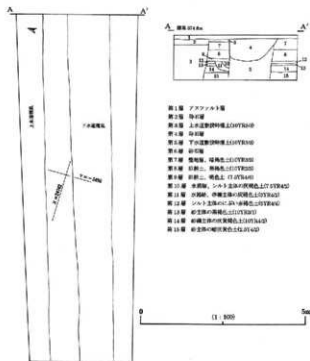
第22図 調査第⑦東区全体図 (1:100)
