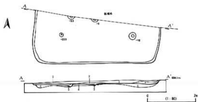
第12図 第11号住居址実測図
