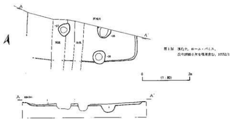
第6图 第2号位层址实测图
