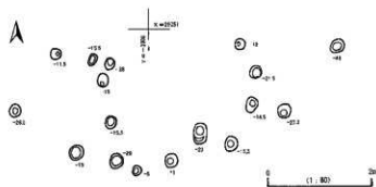
第17図 ピット群実測図
