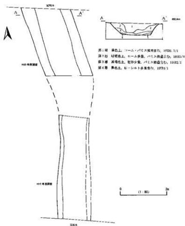
第15図 第4号住居実測図
