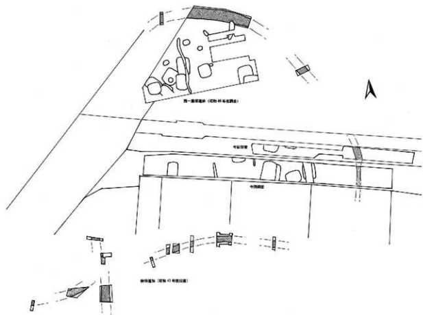
第3図 西一里塚遺跡調査全体図 (1:1,000)
