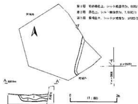
第19図 第1号竖穴遺構実測図
