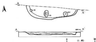
第13図 第12号住居址実測図
