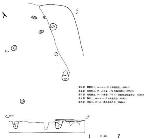
第8図 第4号住居址実測図
