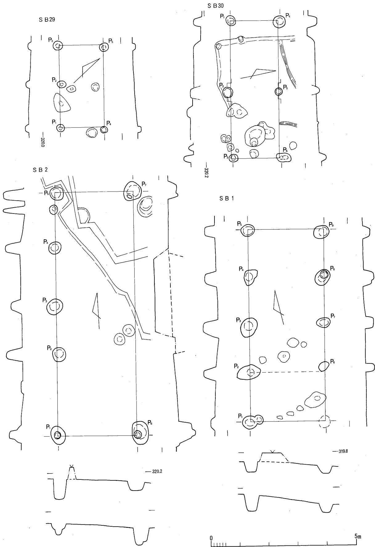
图12 掘立柱建物址 1 : 80
