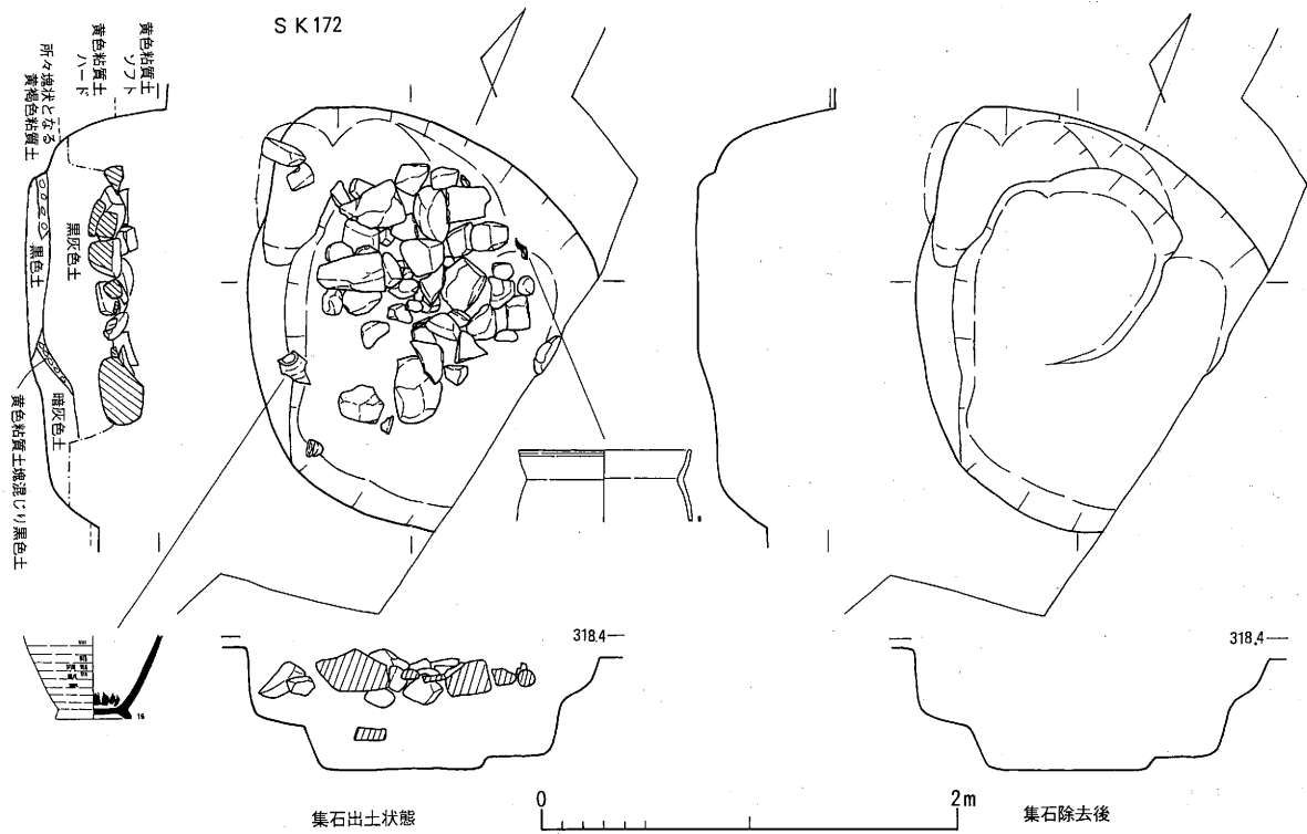
図11 竪穴住居址H35号住居址 1 : 60 土器埋納柱穴 1 : 20 集石土坑S K 172 1 : 40
