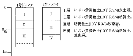
基本層序模式図
