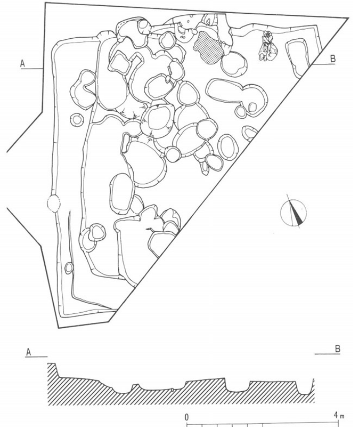
第31図 1号住居跡平面図(1:100)
