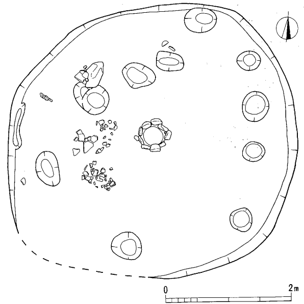
第36図 3号住居跡平面図 (1:60)
