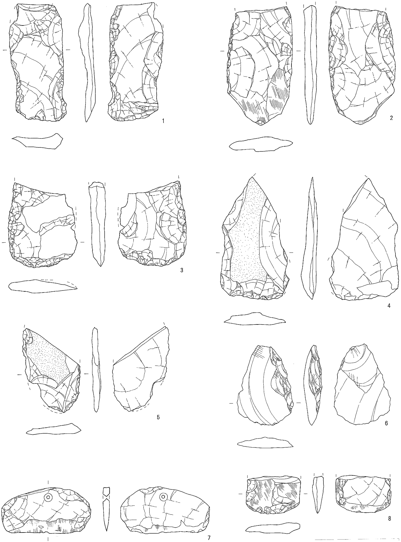
第226图 出土石器实测图〈2〉
