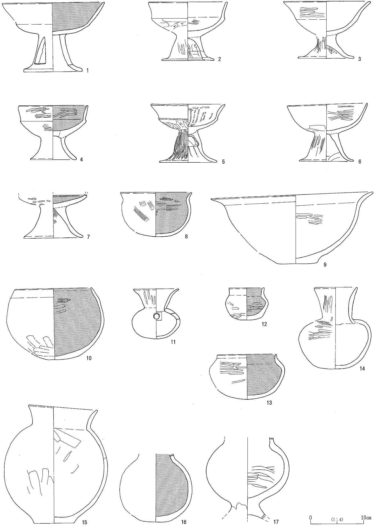
第125图 U t 29号土器集積址出土土器実測図〈2〉
