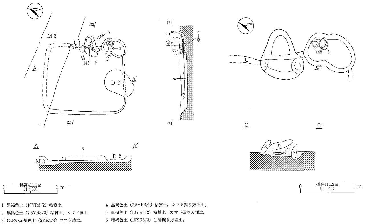
第147図 H 7号住居址カマド掘り方実測図
