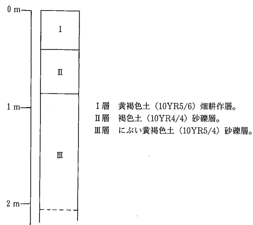
基本層序模式図
