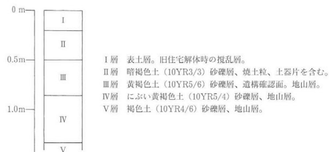
基本層序模式図
