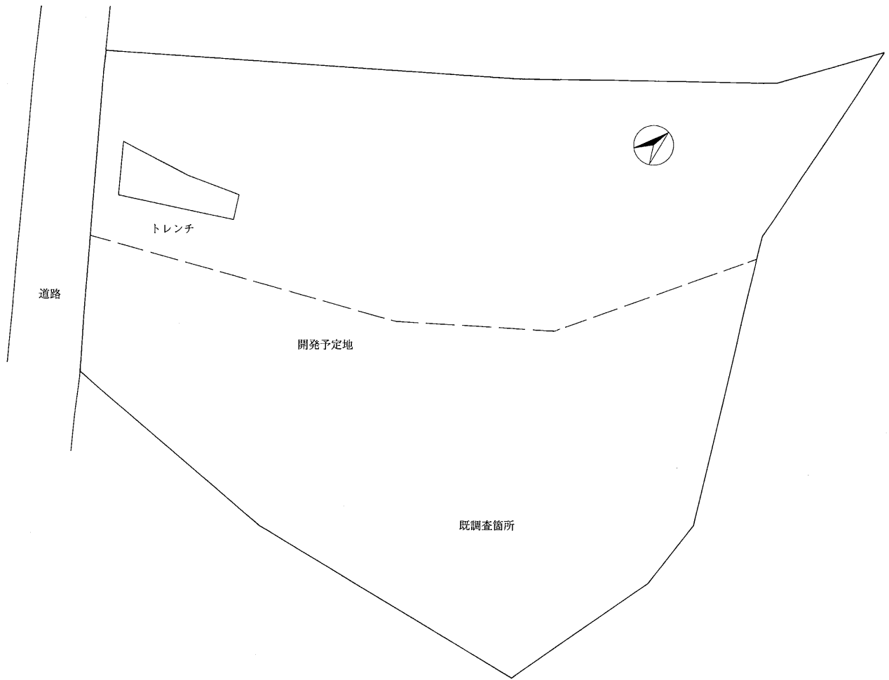
試掘トレンチ設定図 (1 : 500)
