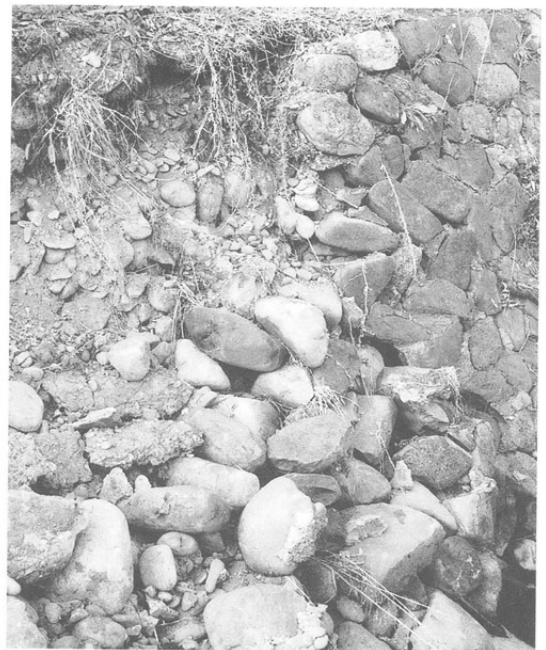
石垣内部の状況（基準番号22の南側）
