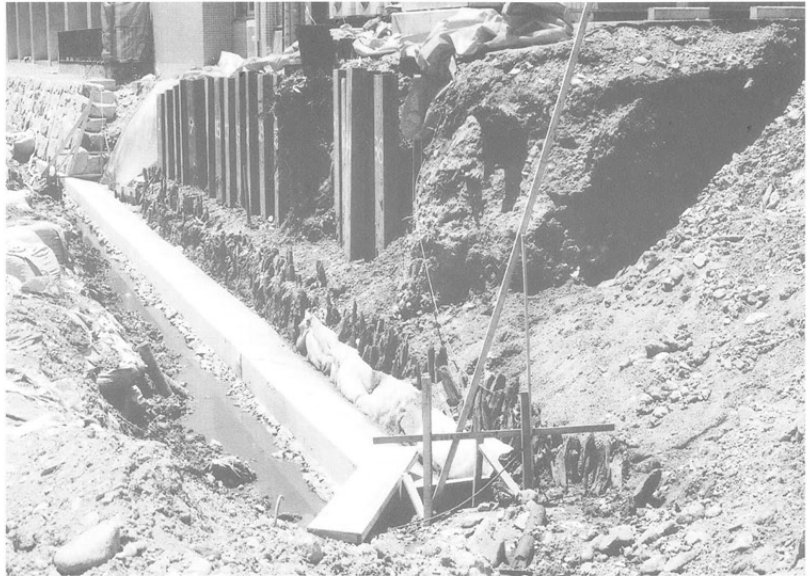
コンクリート布基礎打設状況 (遺構の杭列はこのまま埋め戻した)
