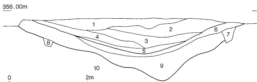
第8図 1号溝跡断面図 (1:60)
