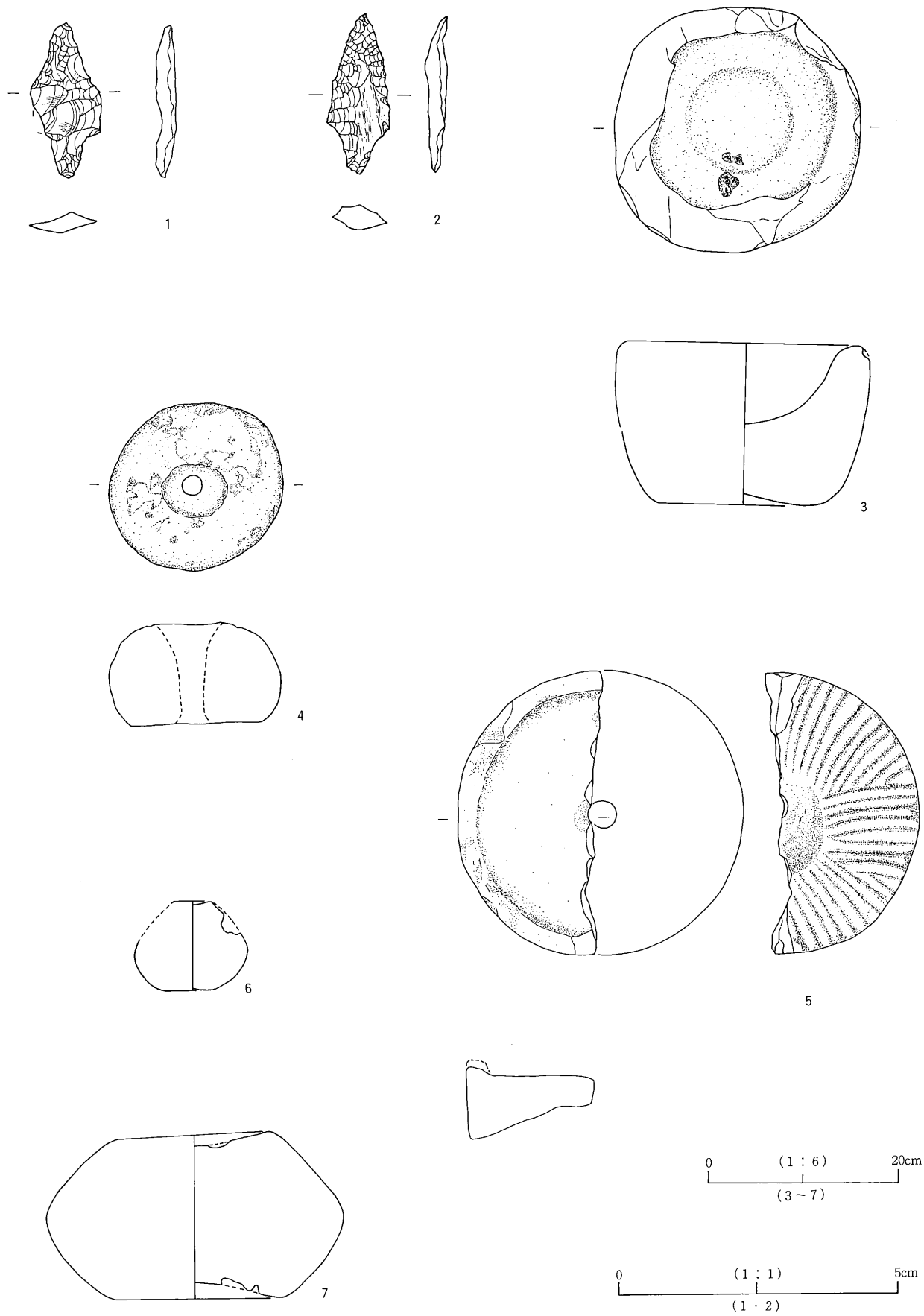
第3图 达山D遺跡出土遺物実測図2
