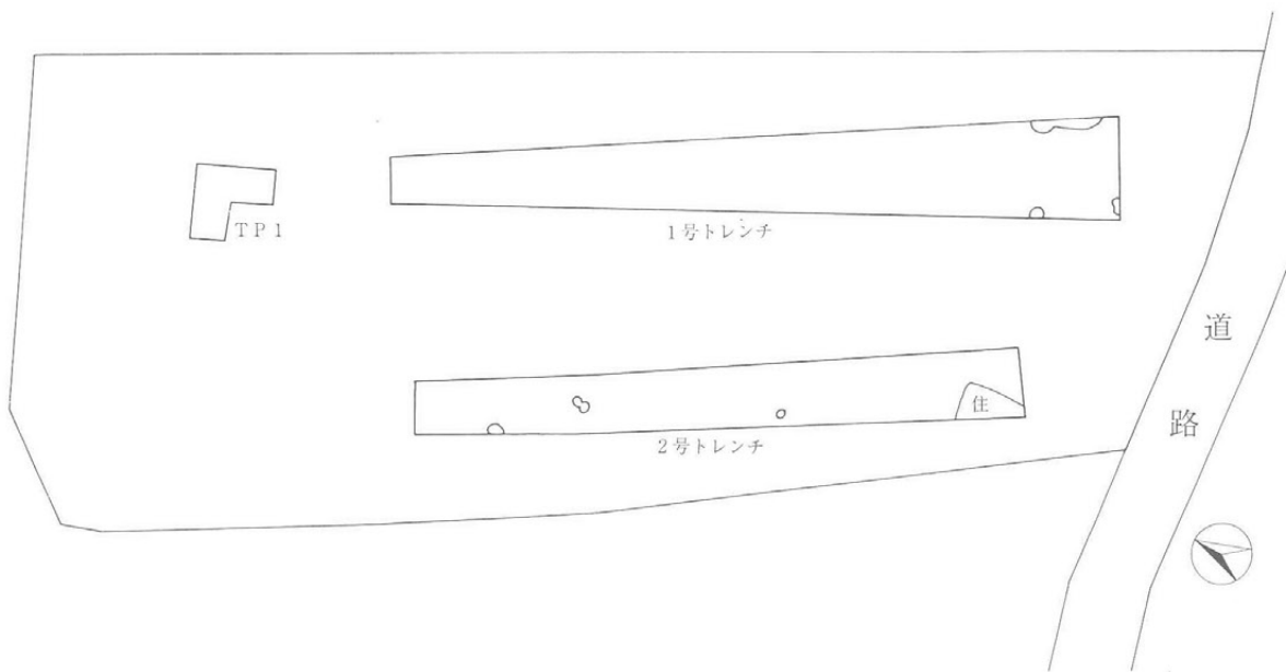
試掘トレンチ設定図 (1:400)
