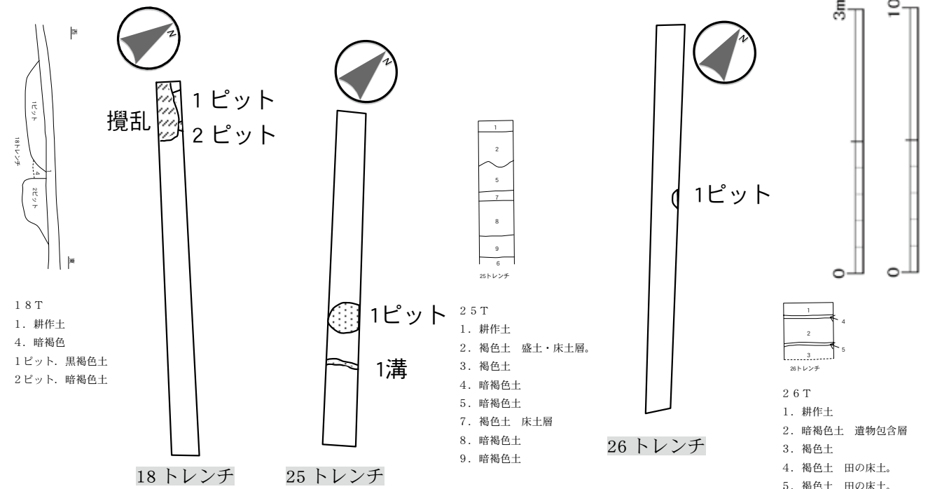
第5図 トレンチ平面図 (1/200)・セクション図 (1/60)
