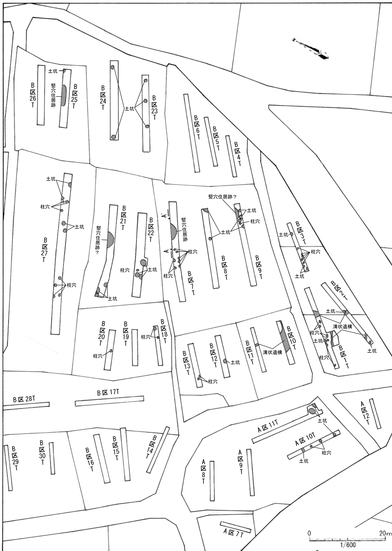
第7図 変電所地点遺構配置図(1) S=1/600
