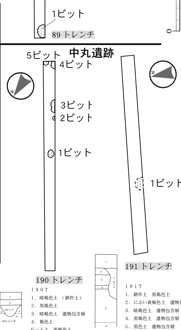
第6図 トレンチ平面図 (1/200)・セクション図 (1/60・1/150)
