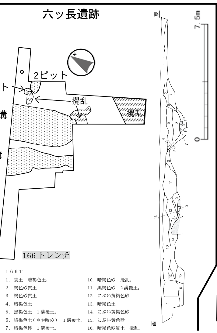
第6図 トレンチ平面図 (1/200)・セクション図 (1/60・1/150)
