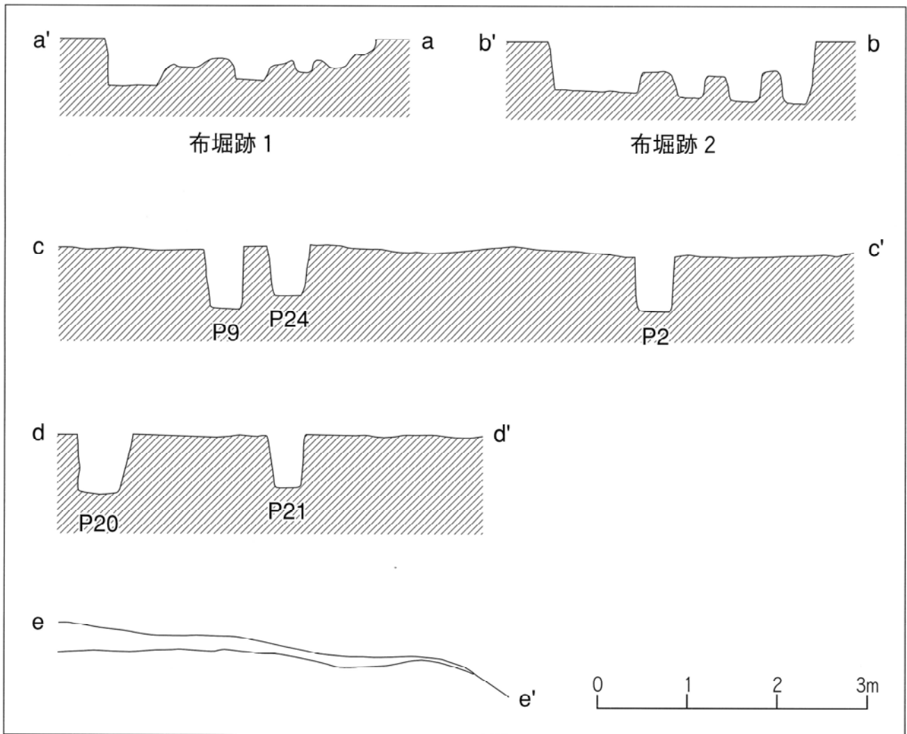
第7図 寺屋敷上部発掘区断面図
