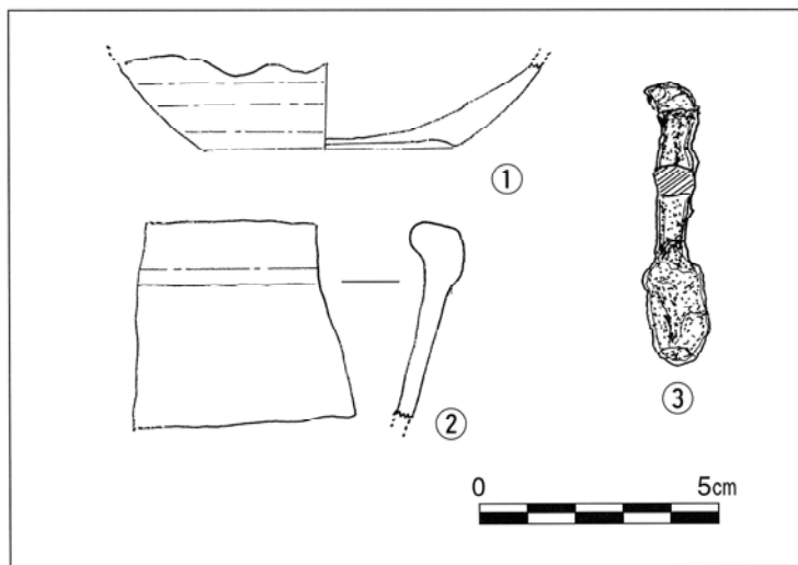
第8図 寺屋敷上部曲輪出土遺物実測図
