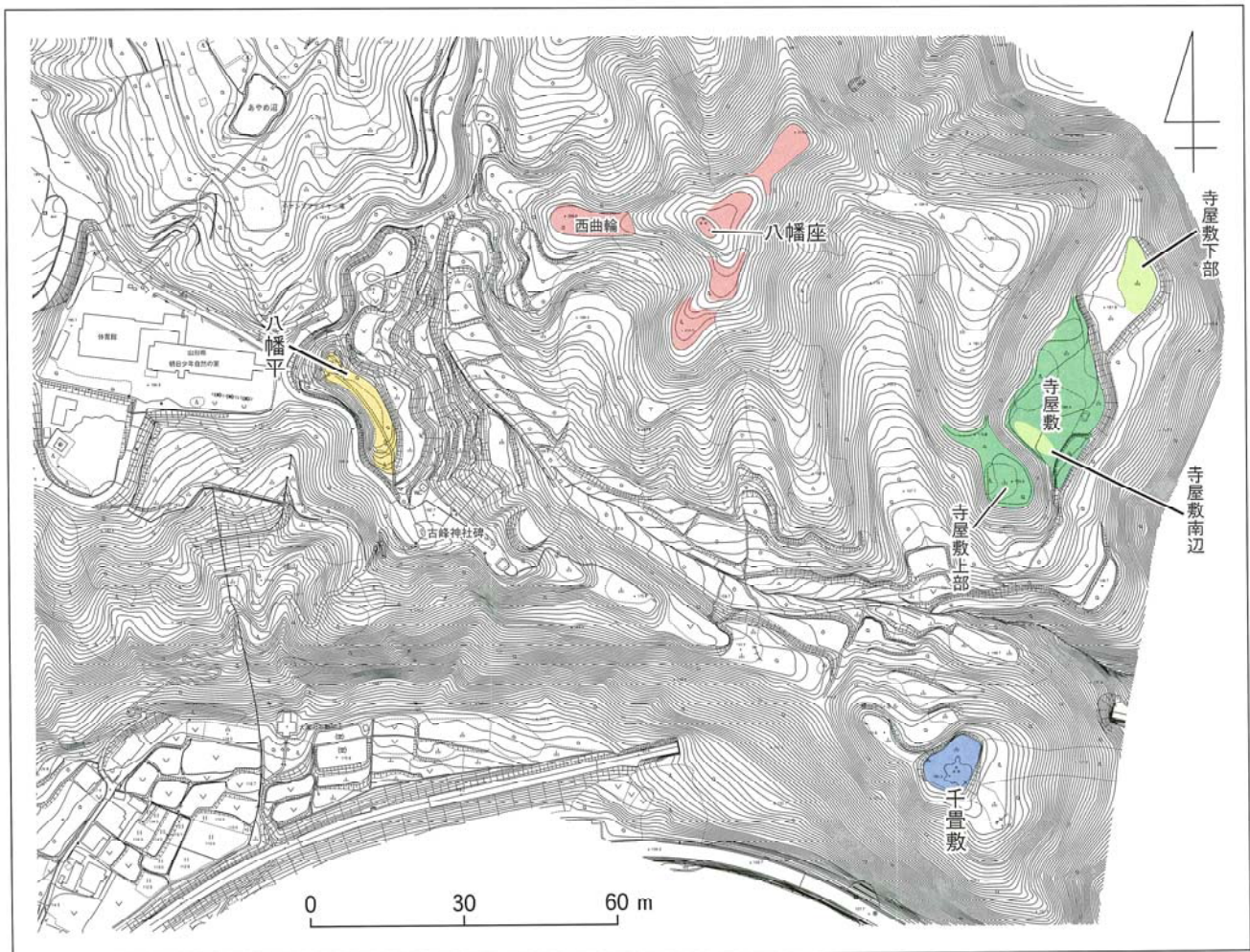
第1図 左沢楯山城全体図
