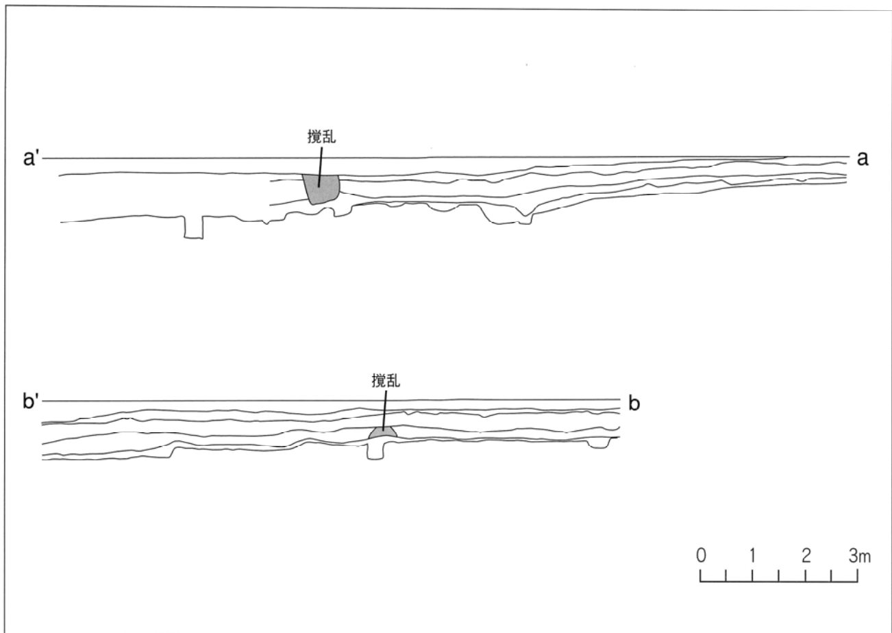
第10図 寺屋敷トレンチ断面図
