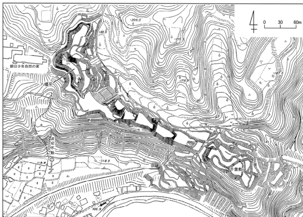
第13図 八幡平曲輪周辺図
