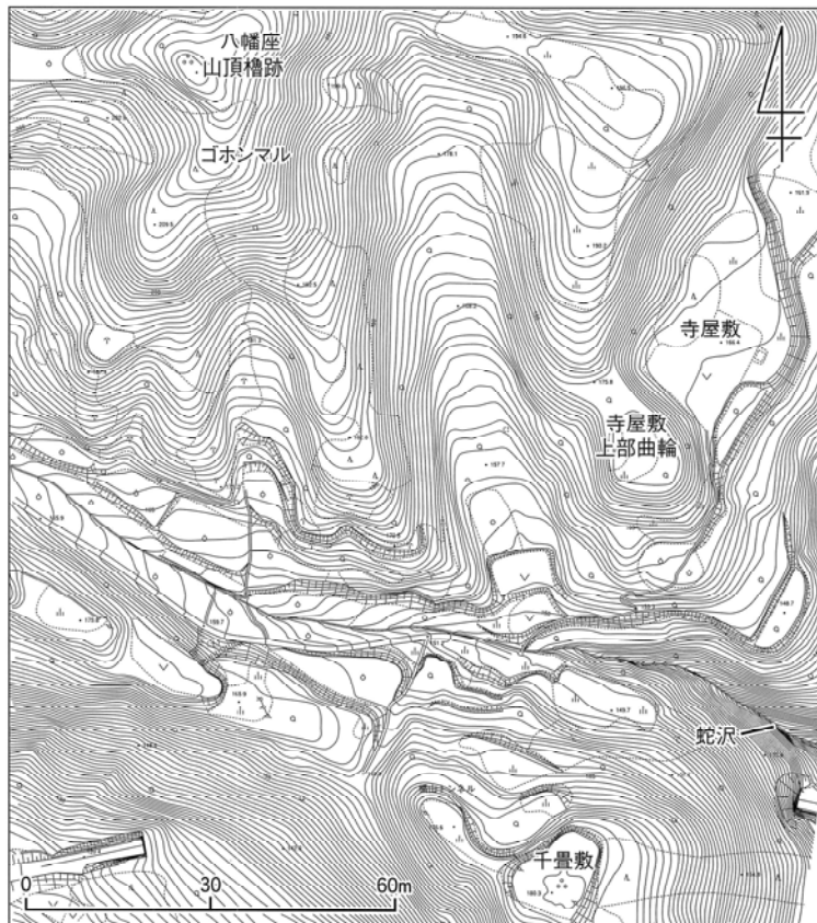
第4図 寺屋敷上部 曲輪周辺図
