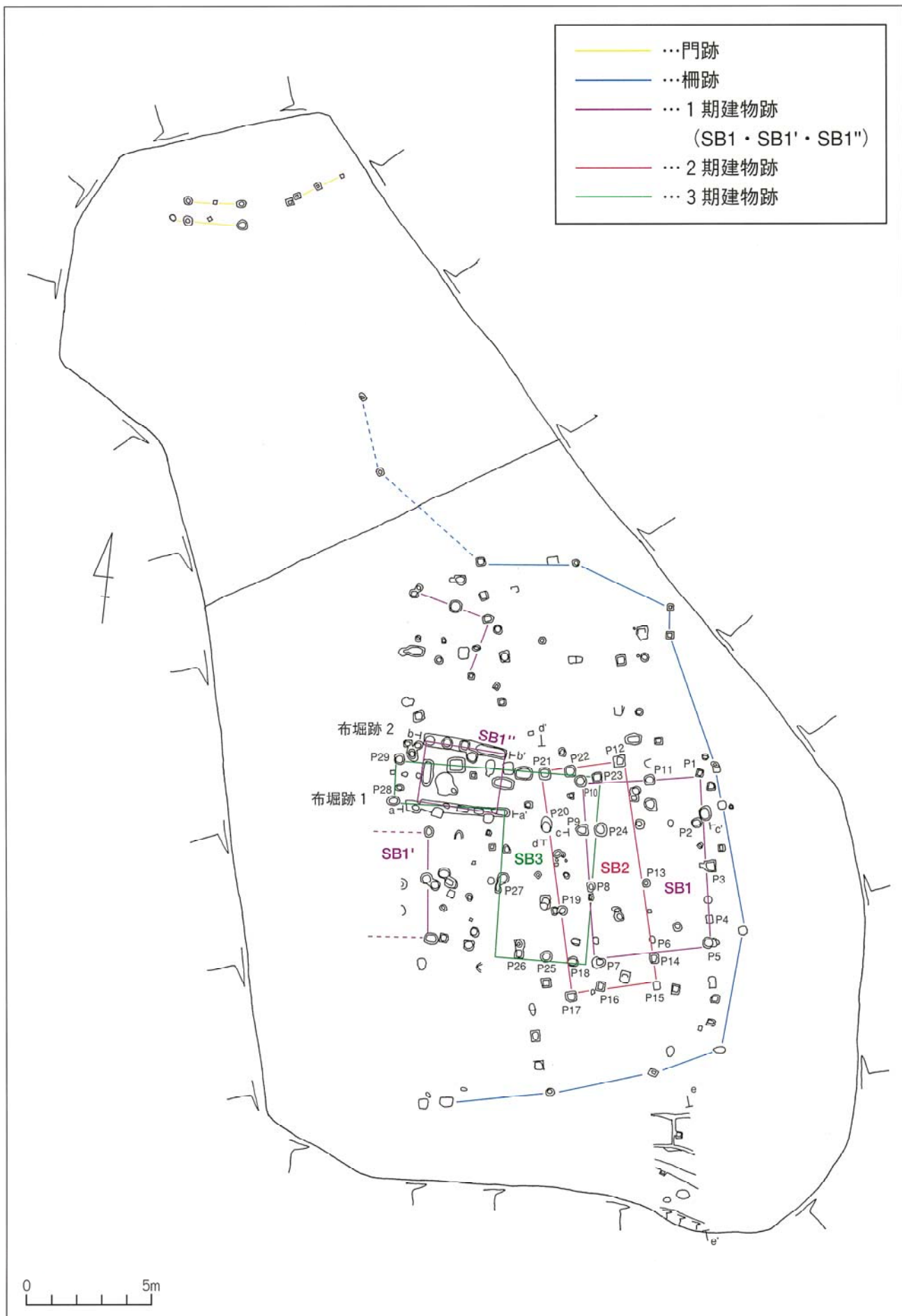
第 6 図 寺屋敷上部遺構配置図
