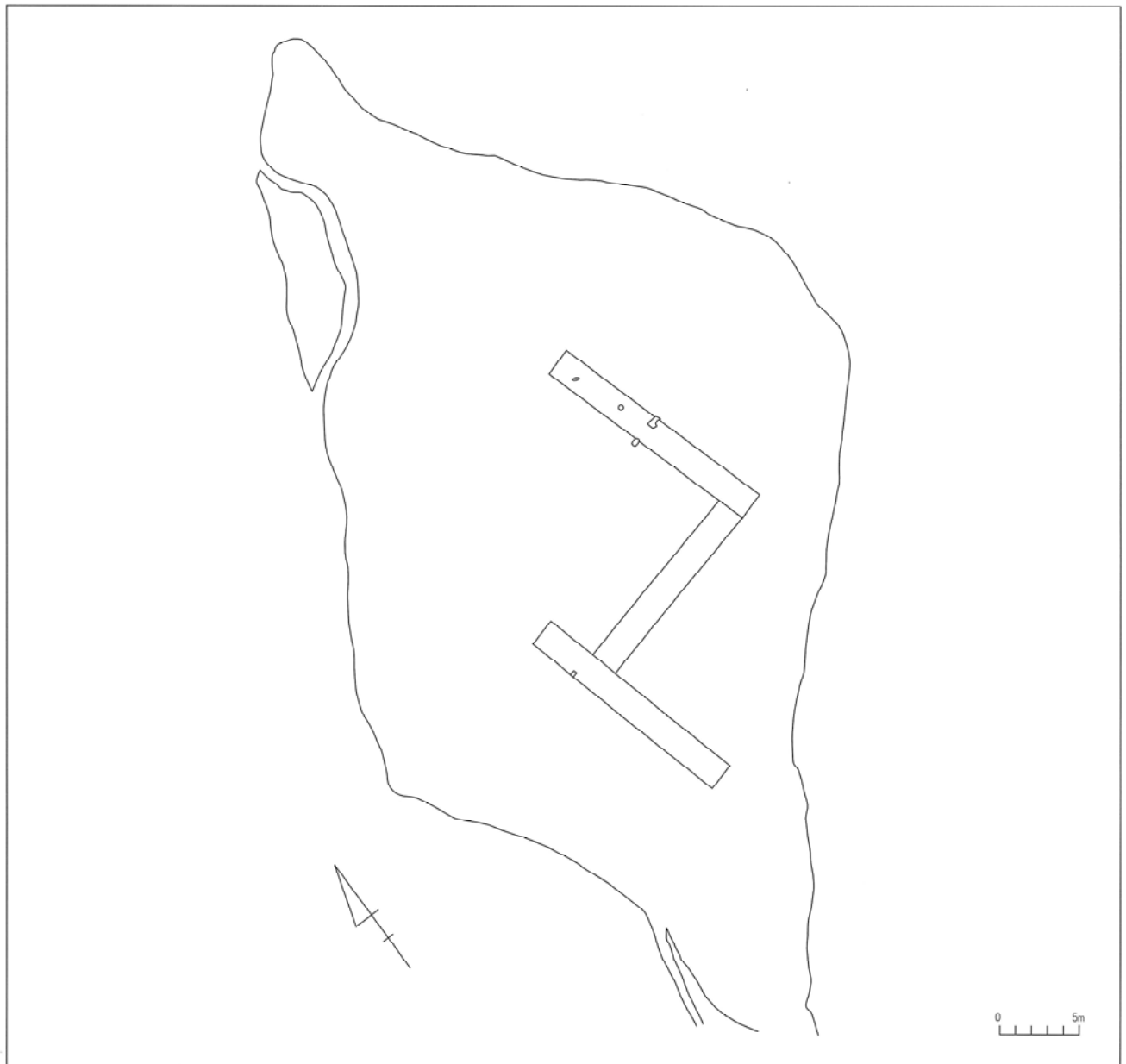
第11図 寺屋敷下部曲輪トレンチ設定図
