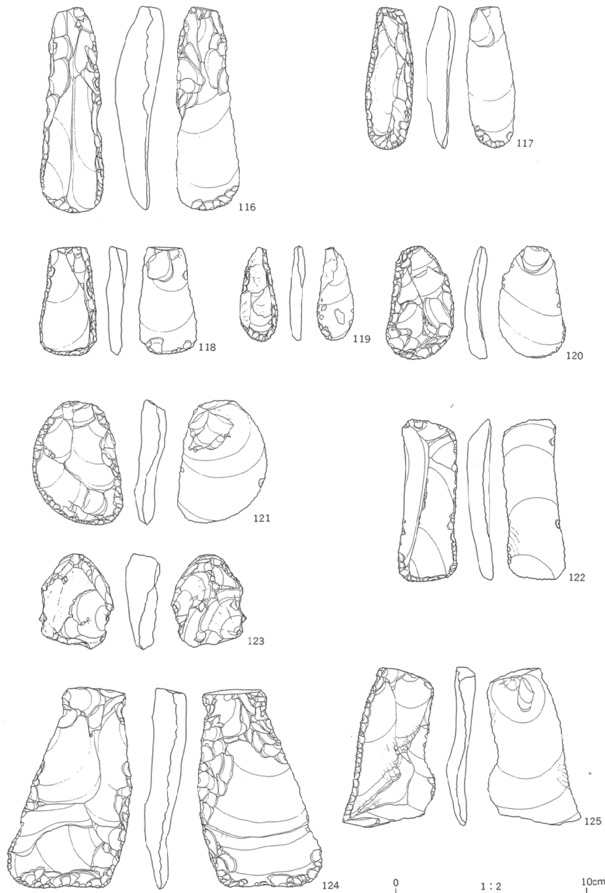
第88図 石器実測図 搔器・削器
