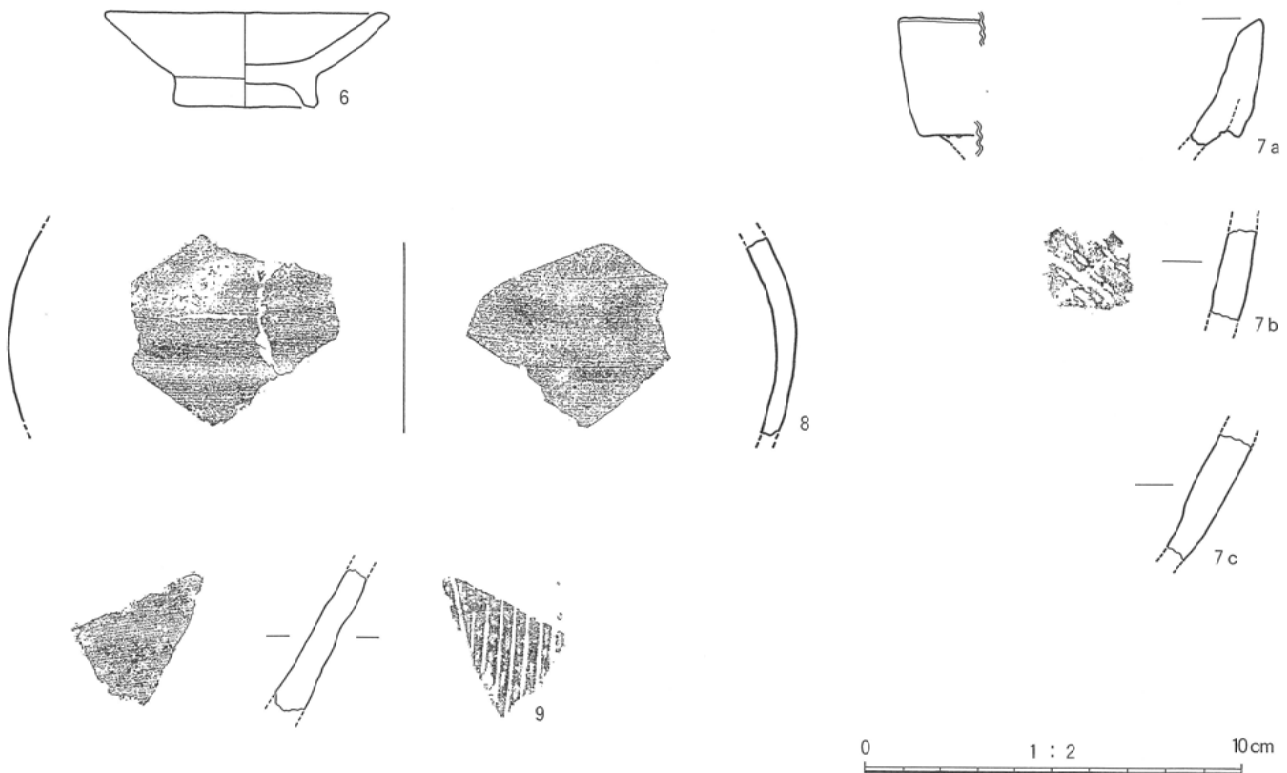
第13図 遺物実測図4（第Ⅲ類土器他）
