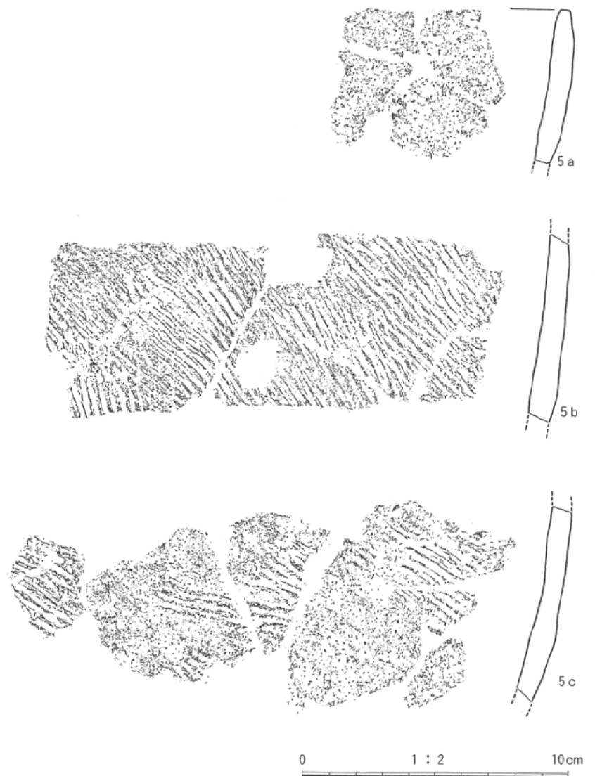
第12図 遺物実測図3（第Ⅱ類土器）
