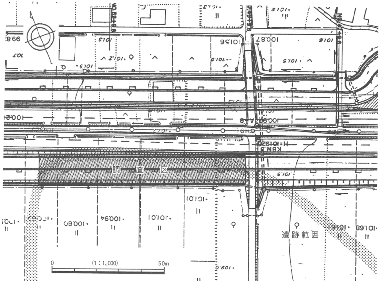
第1図 調査区概要図
