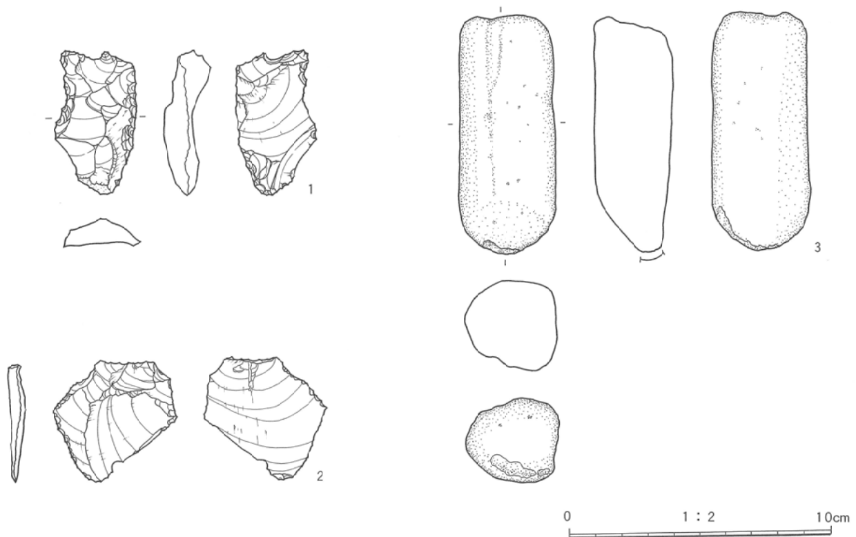
第9図 遺物実測図1（石器）
