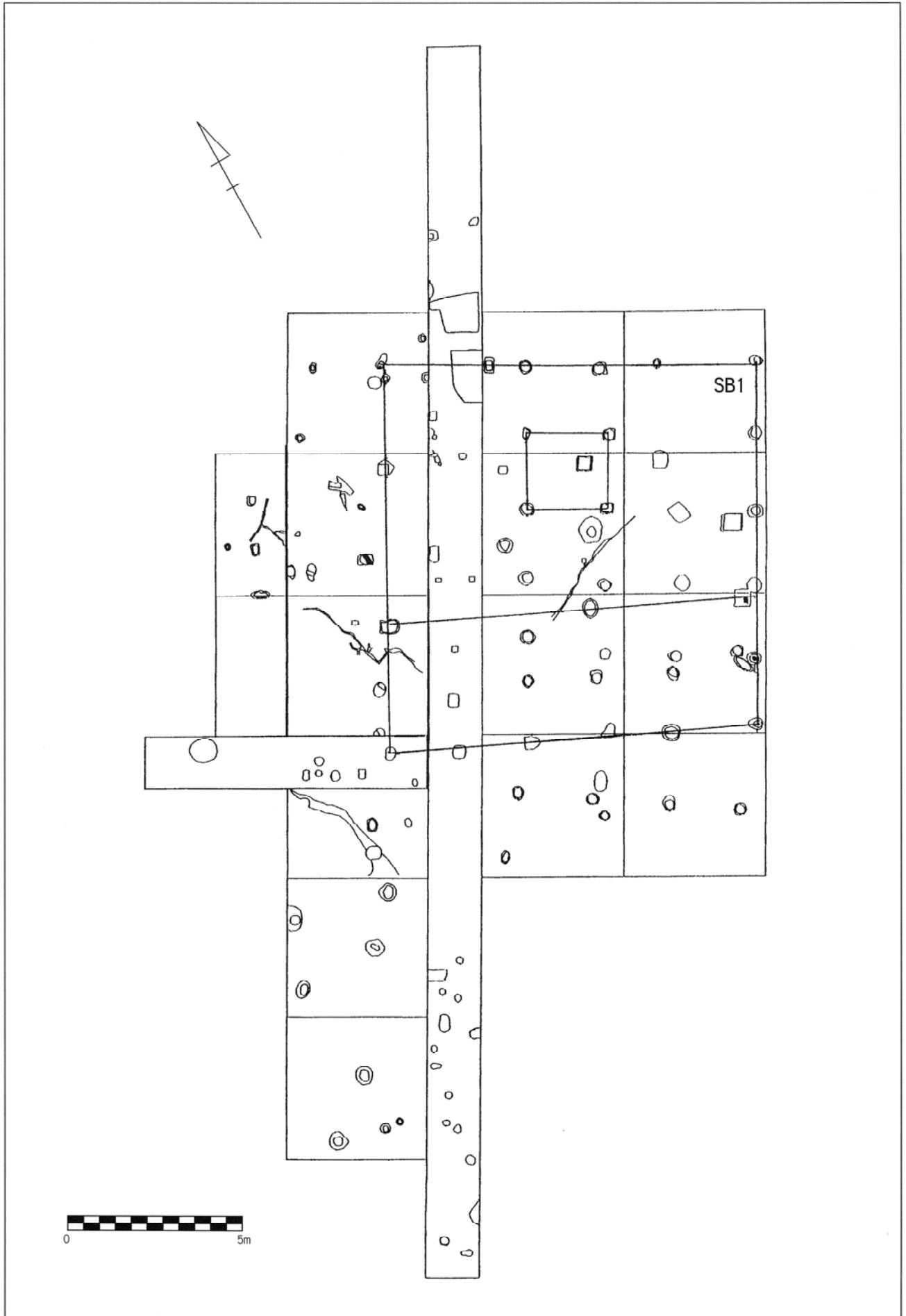
第6図 寺屋敷遺構配置平面図
