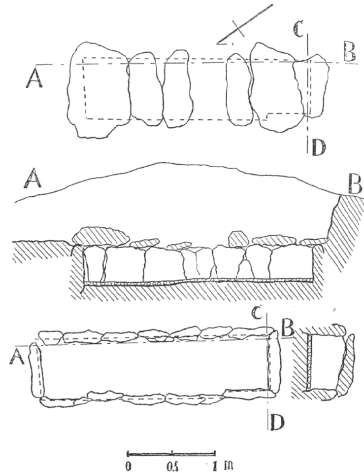
第10図 高原古墳石棺実測図
