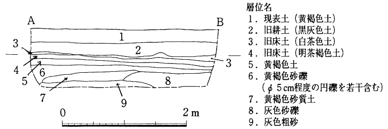
第19図 池浦遺跡 第1地点 北壁断面図
