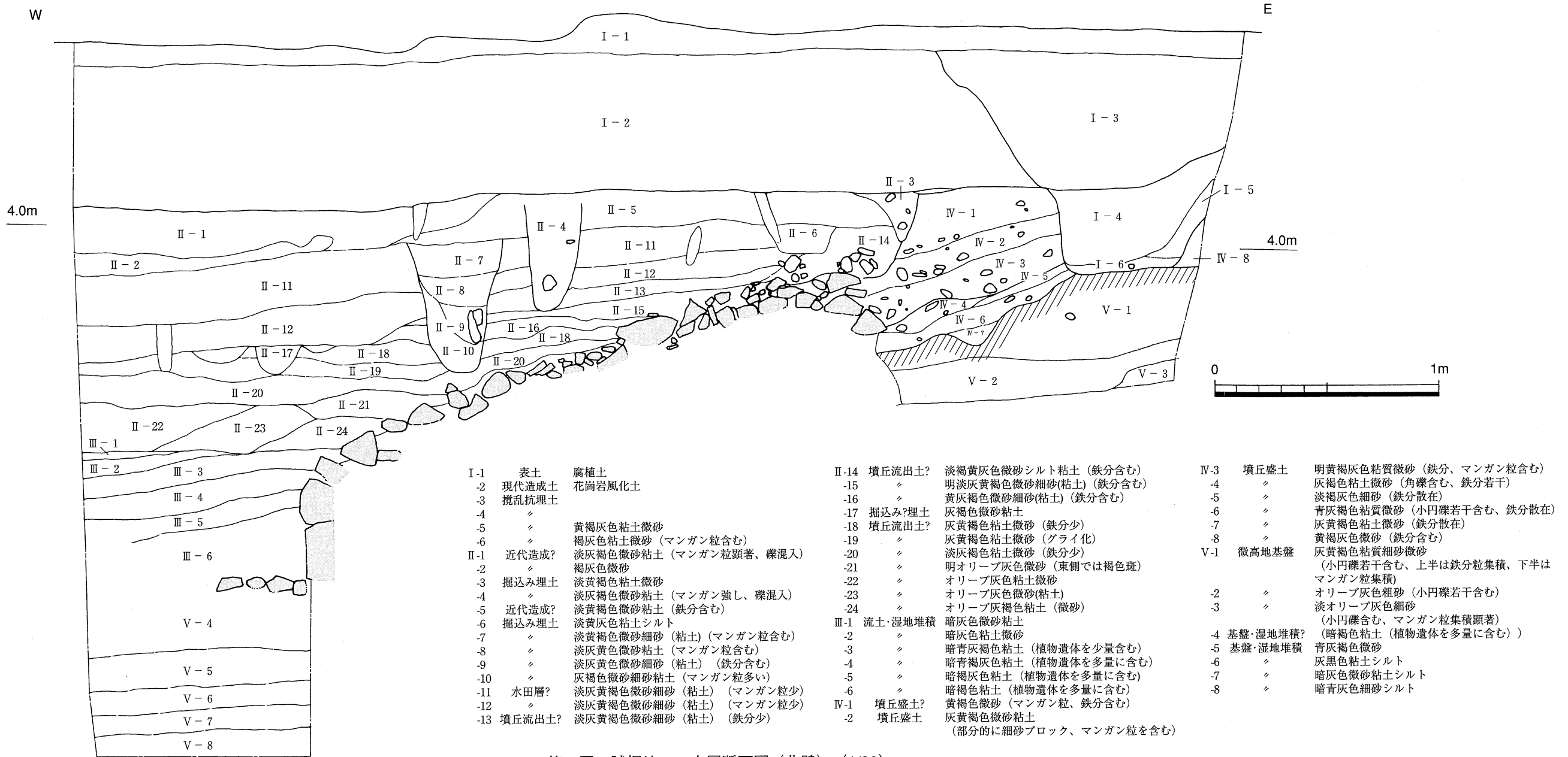
第7図 試掘坑I・土層断面図(北壁) (1/20)
