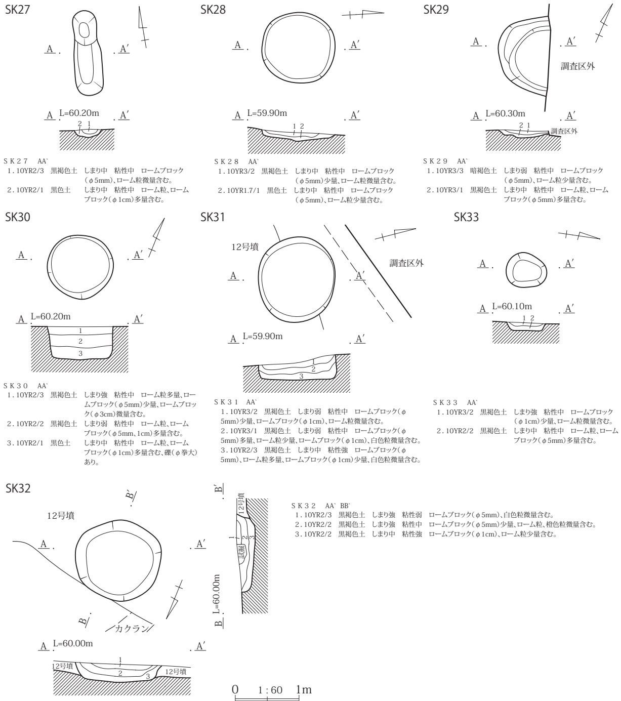
第 18 図 27～33 号土坑平面図・断面図
