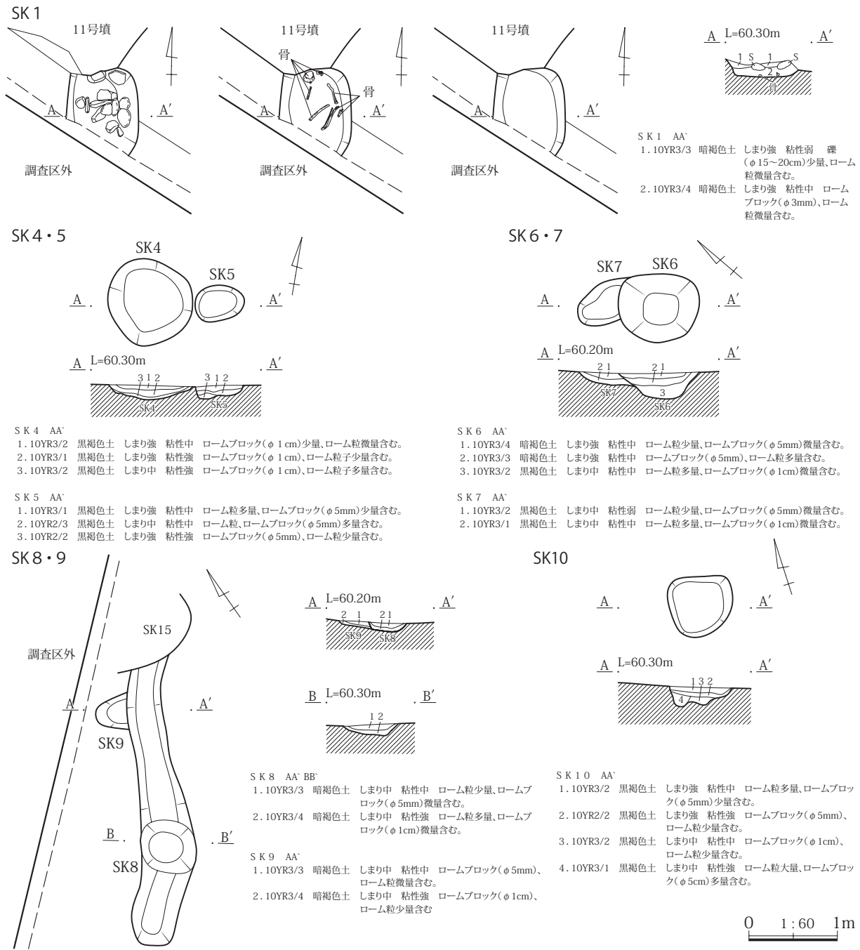
第 13 図 1・4～10号土坑平面図・断面図
