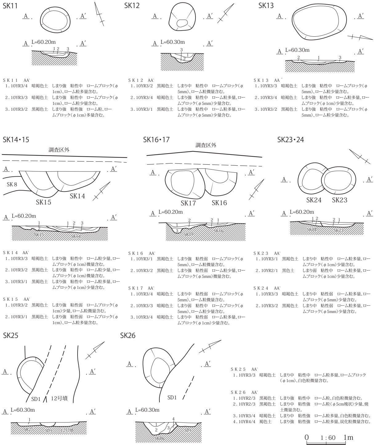
第15図 11～17・23～26号土坑平面図・断面図
