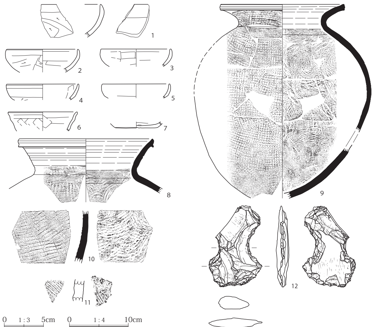
第10図 杉ノ根 12号墳出土遺物実測図
