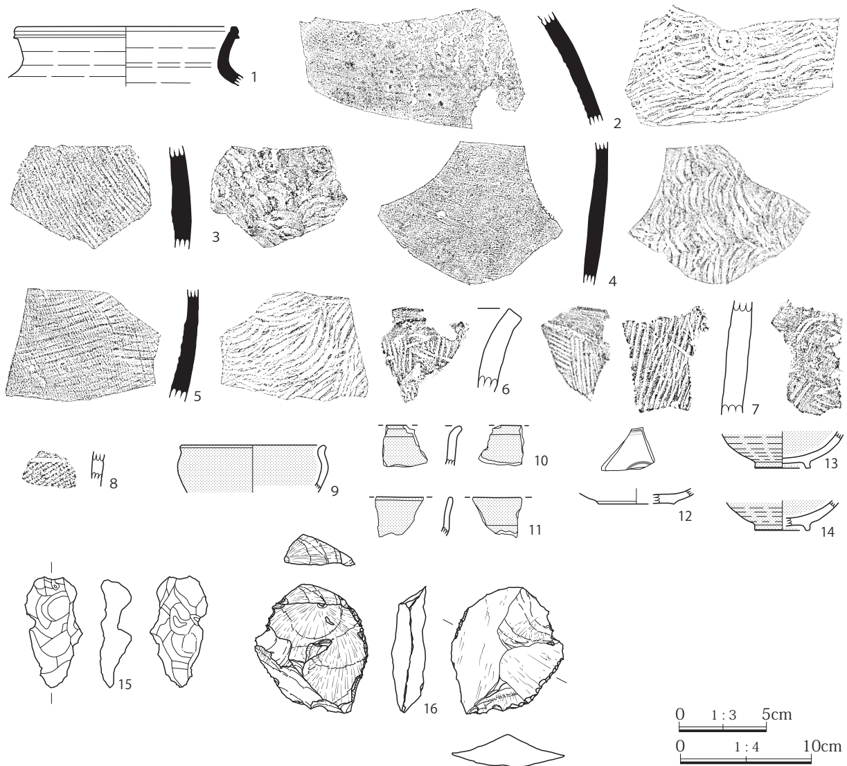
第6図 杉ノ根1号墳出土遺物実測図
