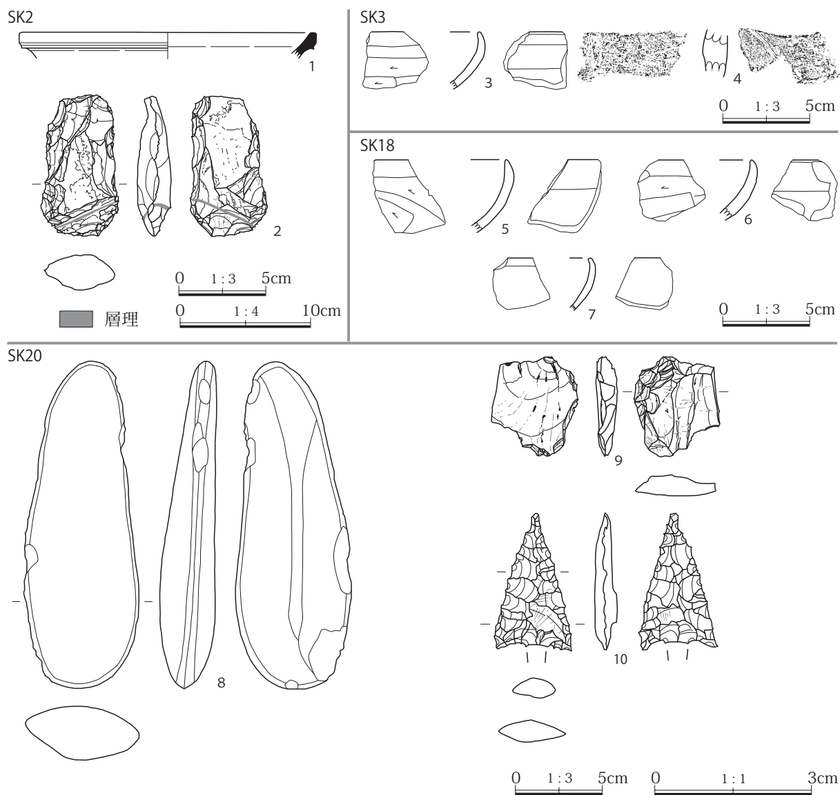
第 19 図 土坑出土遺物実測図
