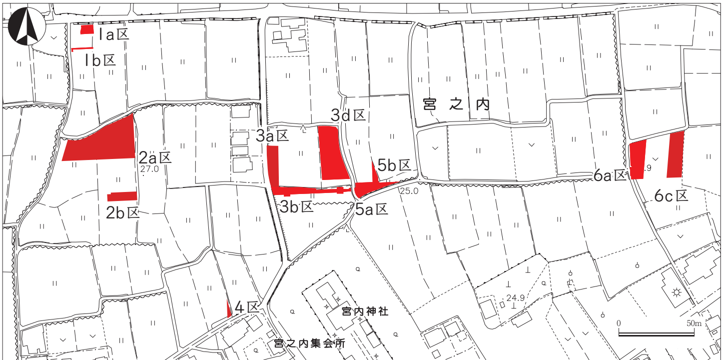
調査区位置図
