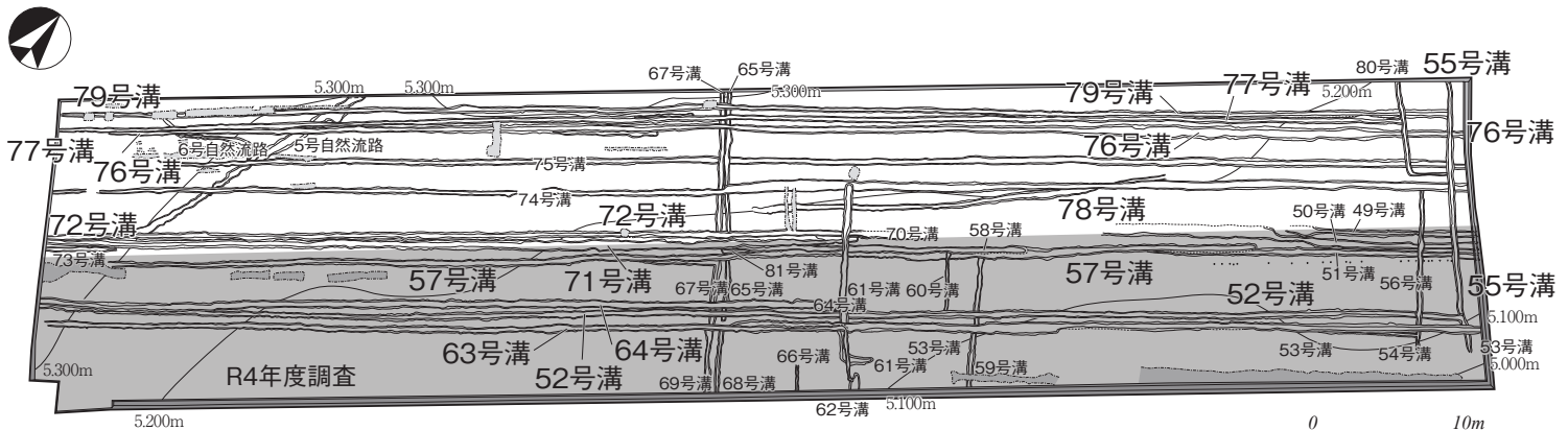
3区 遺構配置図
