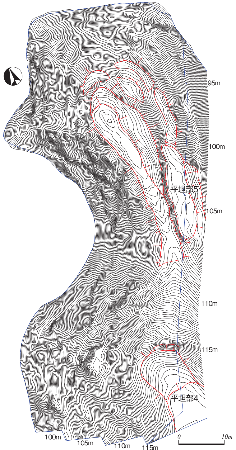
調査前地形測量図
