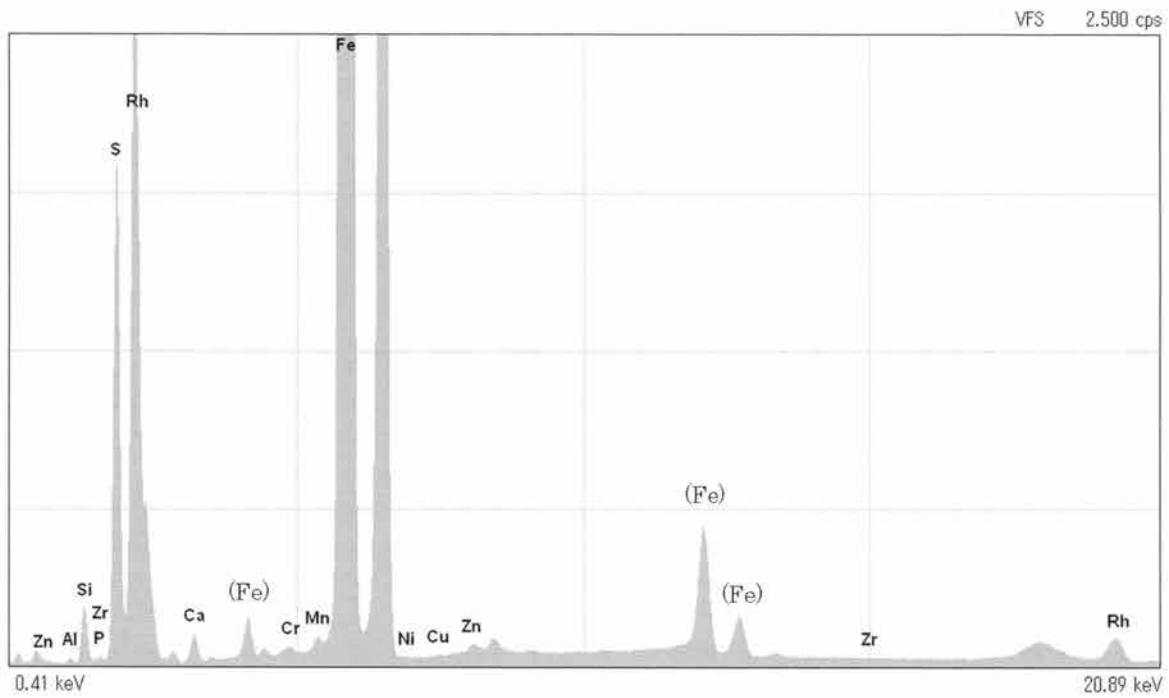
図版2. 磬裏面の鉄Feマッピング測定結果 (スペクトル図は、範囲bのマッピングによる)
