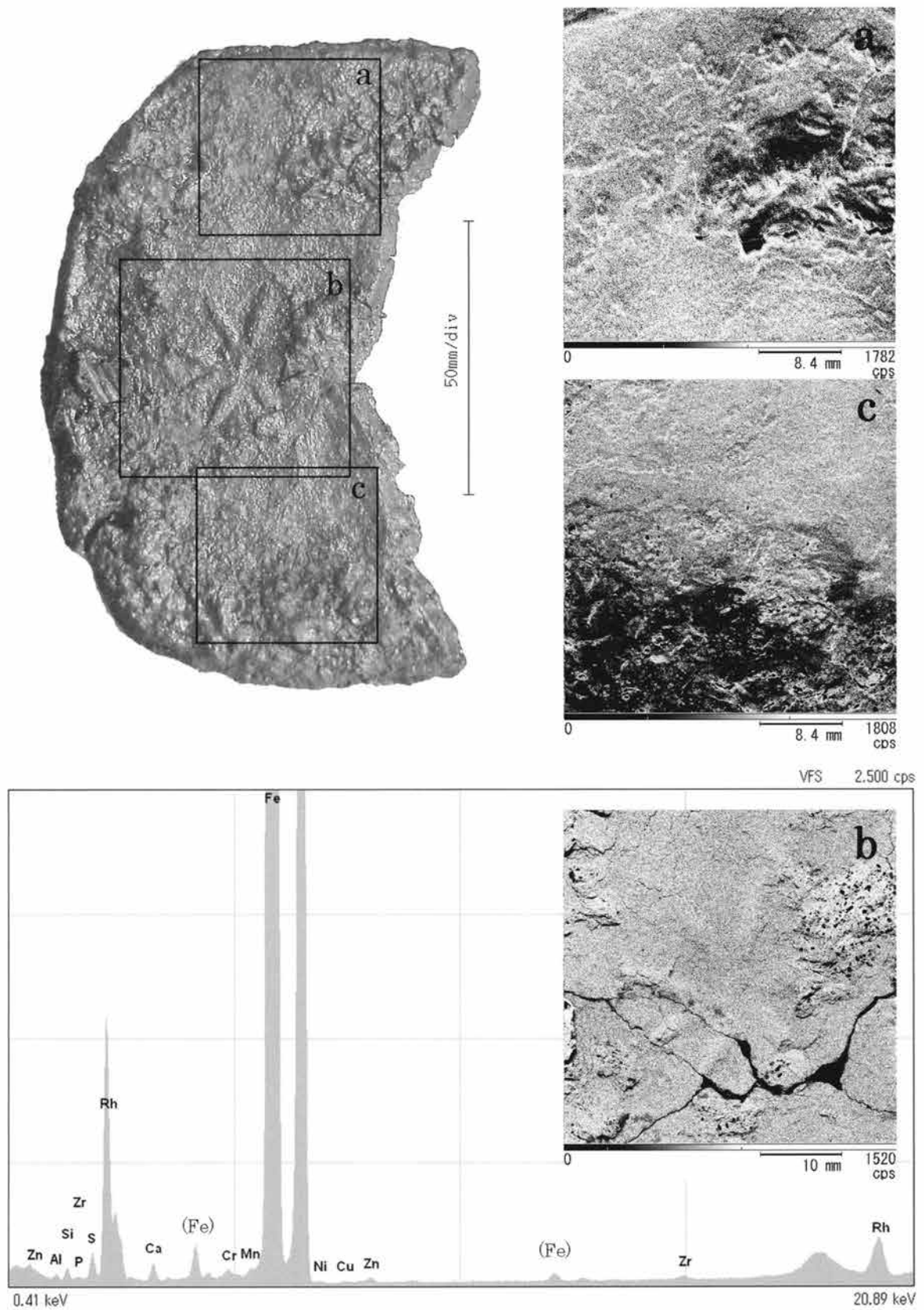
図版1. 礬表面の鉄Feマッピング測定結果 (スペクトル図は、範囲aのマッピングによる)
