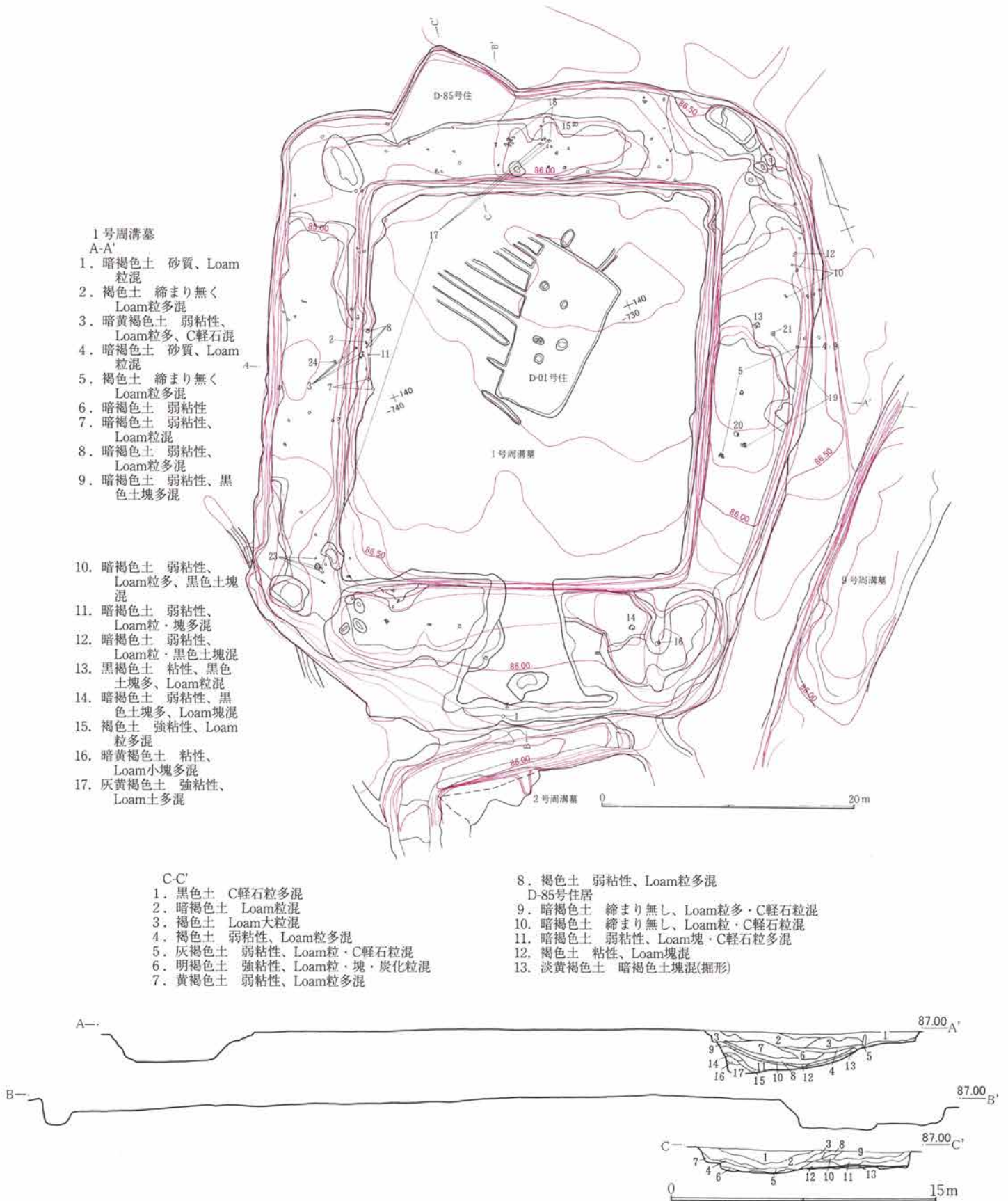
第512図 1号周溝墓
