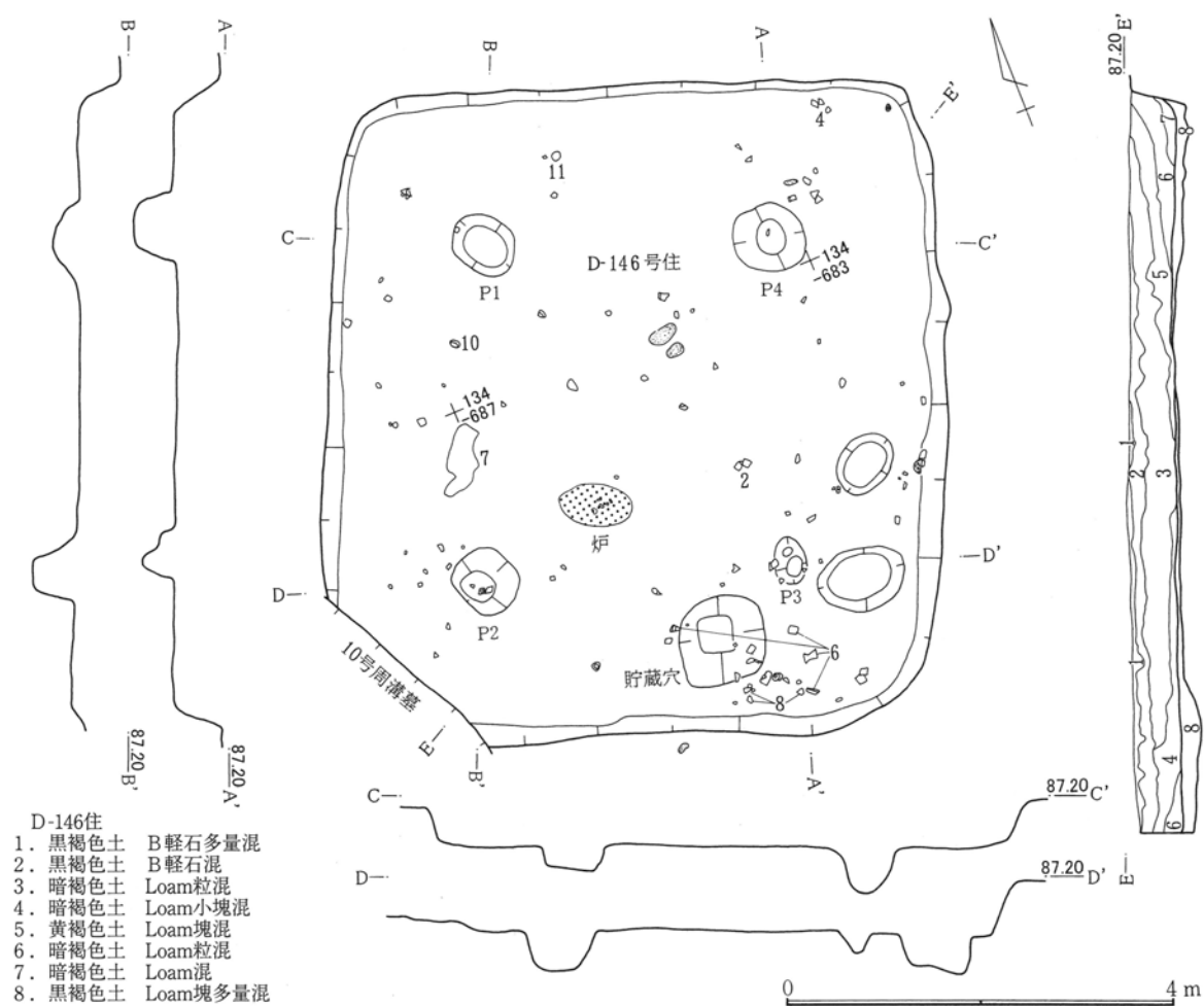
第293図 D-146号住居跡
