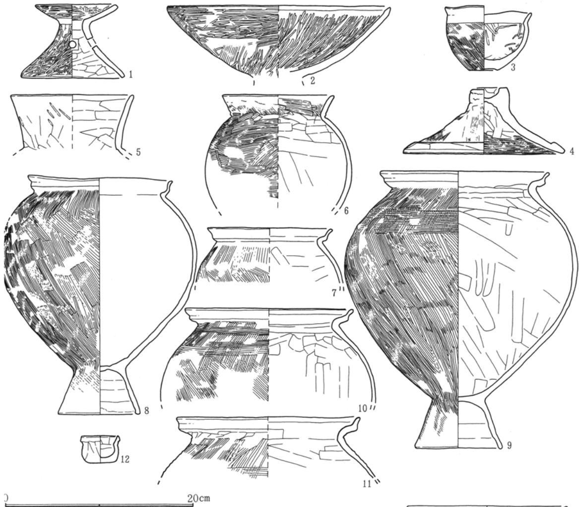
第459図 D-160号住居跡出土遺物
