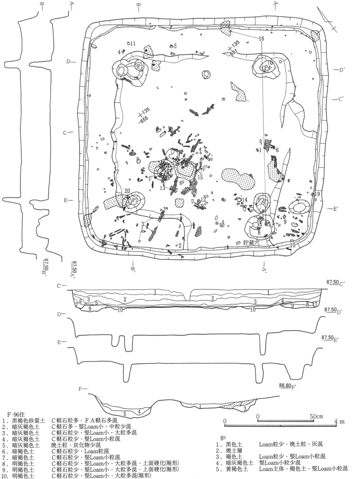
第340図 F-96号住居跡
