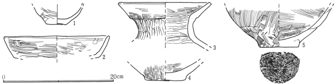
第509図 工境-12号住居跡出土遺物
