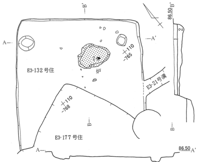
第308図 E 3 -132号住居跡
