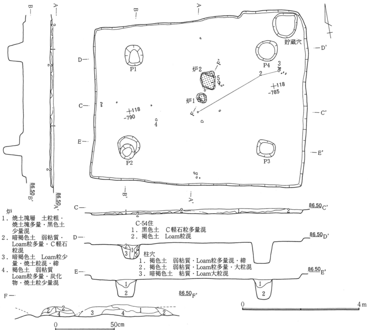
第246図 C-54号住居跡
