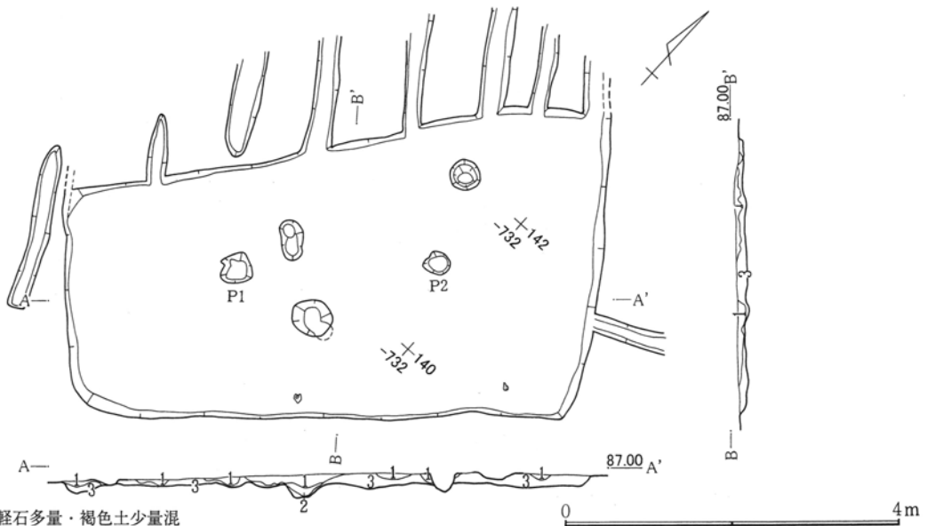
第249図 D-01号竪穴跡
