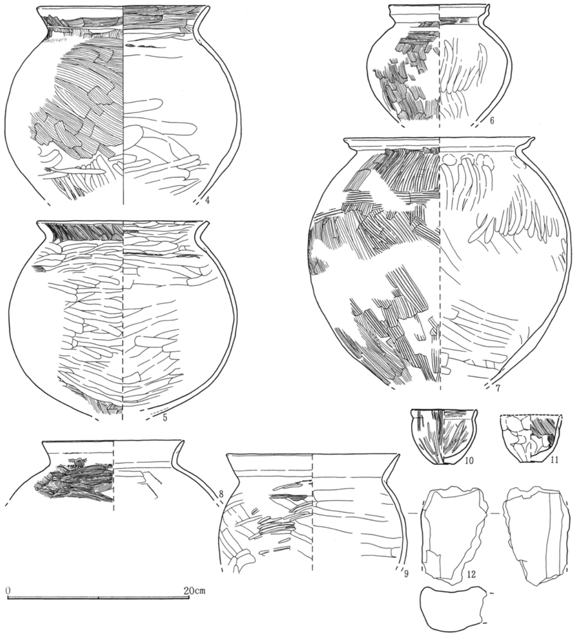
第390図 A 1 -49号竪穴跡出土遺物（2）
