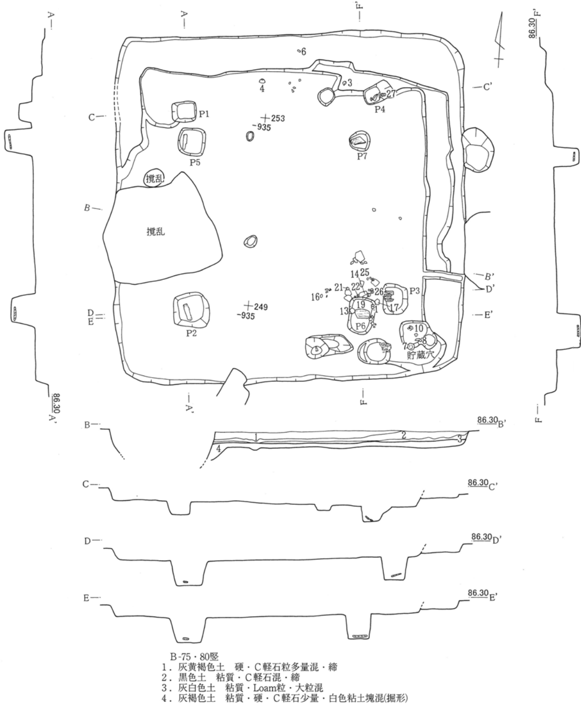
第238図 B-75号堅穴跡
