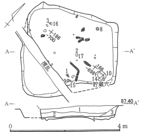
D 3 -15竪 1. 暗褐色土 C軽石・鉄分土混 2. 暗褐色土 3. 黒褐色土 Loam混土 4. 黒褐色土 砂質・Loam塊多量混 第261図 D 3 -15号竪穴跡
