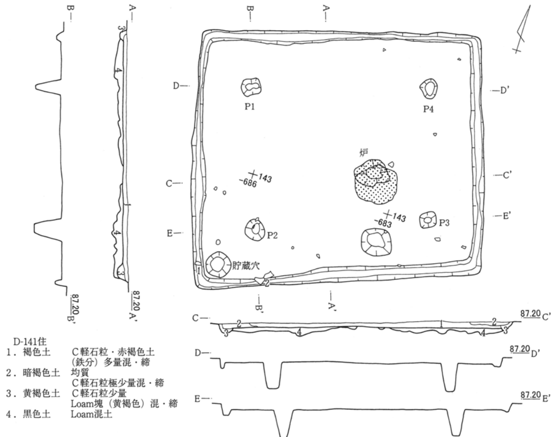
第289図 D-141号住居跡
