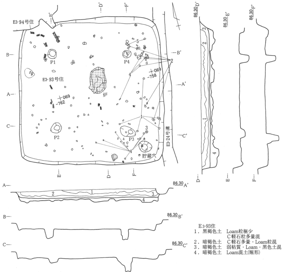
第302図 E 3 -93号住居跡
