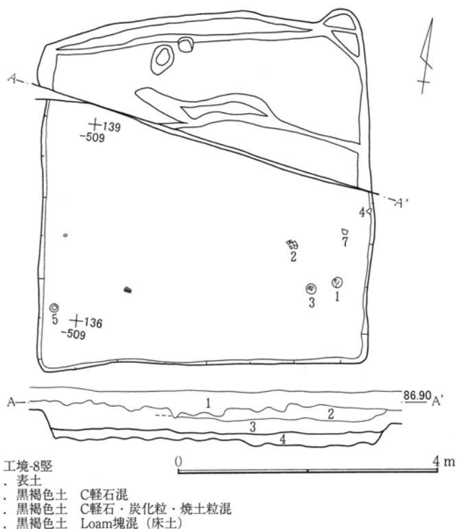
第348図 工境-8号竪穴跡
