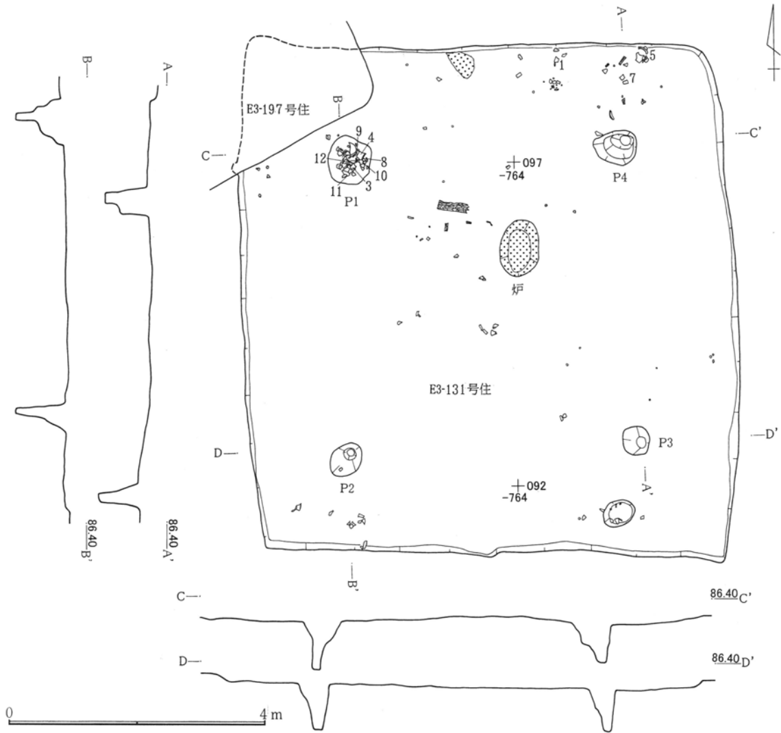
第307図 E 3 -131号住居跡
