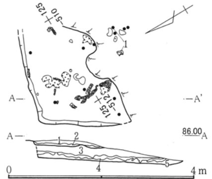
第343図 G-98号竪穴跡
