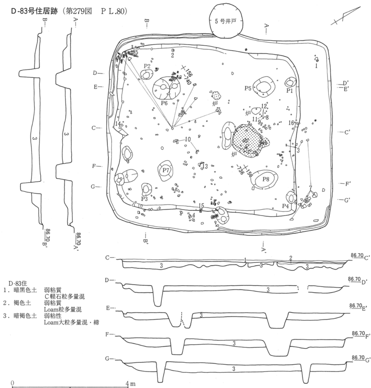
第279図 D-83号住居跡
