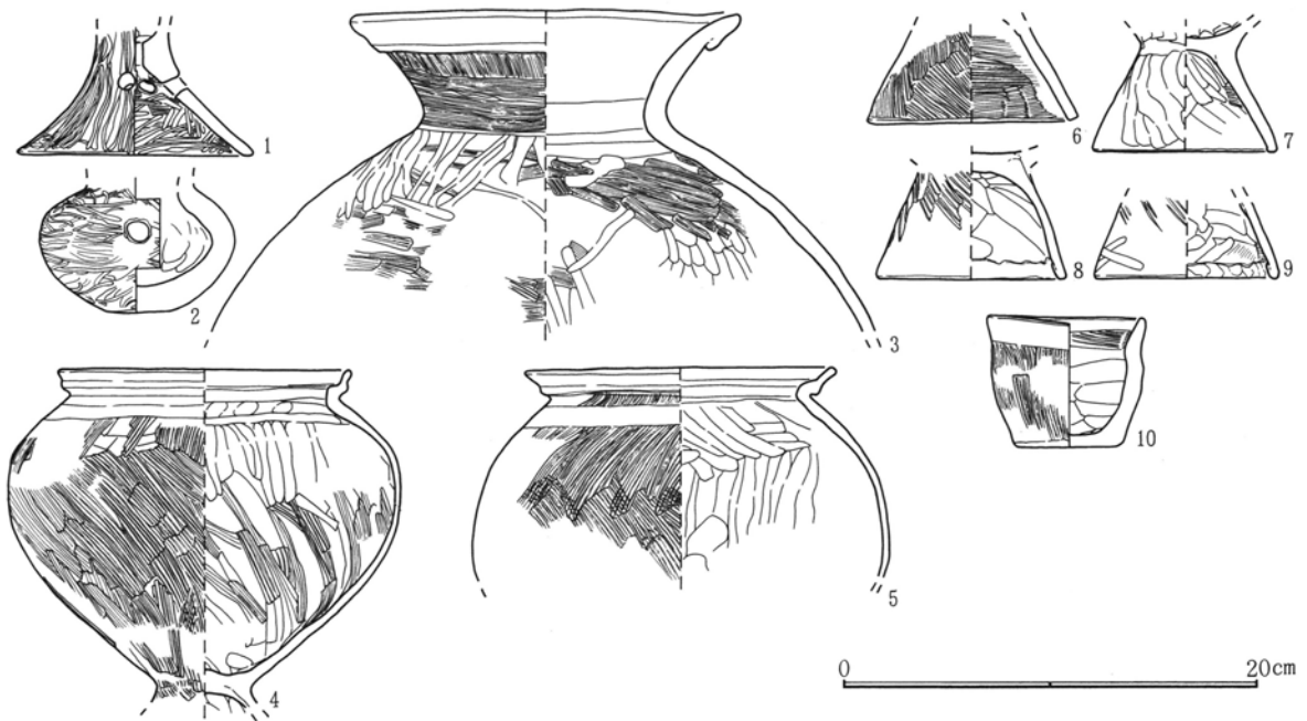
第381図 A1-28号住居跡出土遺物
