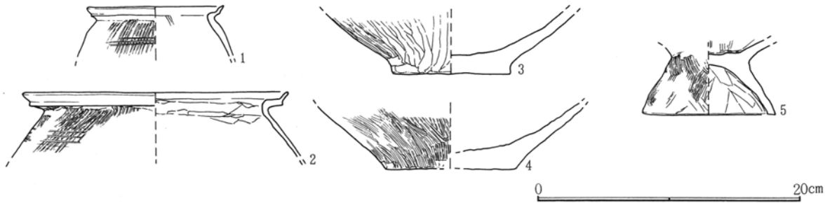
第443図 D 3 -38号住居跡出土遺物
