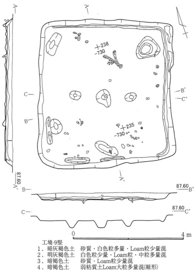
第349図 工境-9号竪穴跡
