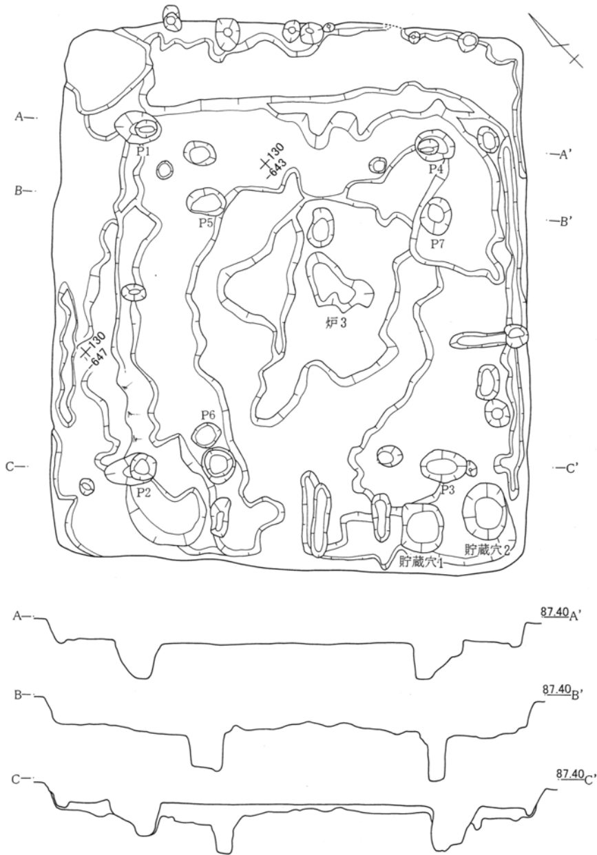
第338図 F-92・93号住居跡掘形
