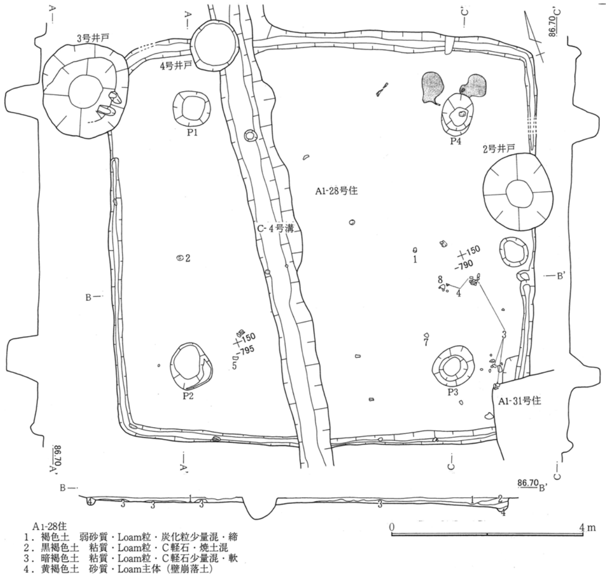
第219図 A1-28号住居跡
