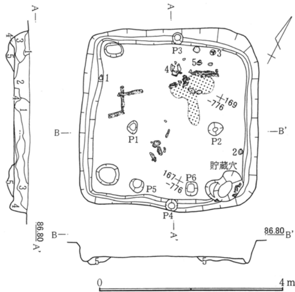
第214図 A1-19号住居跡
