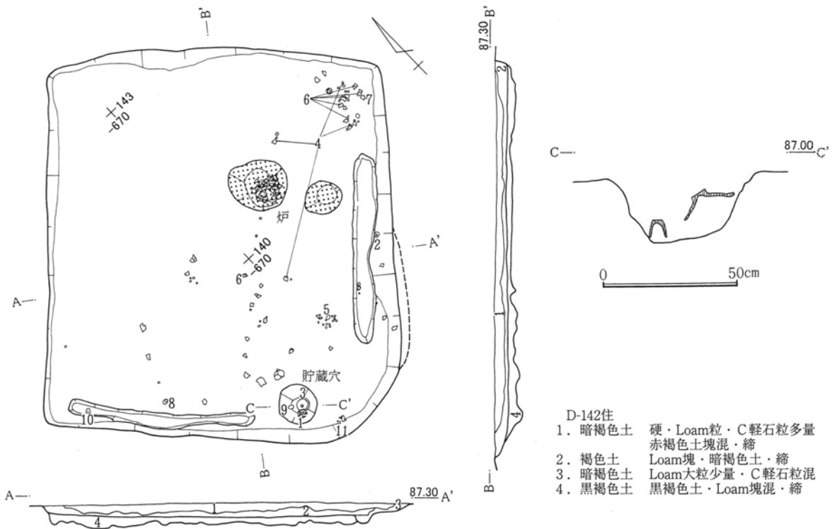
第290図 D-142号住居跡
