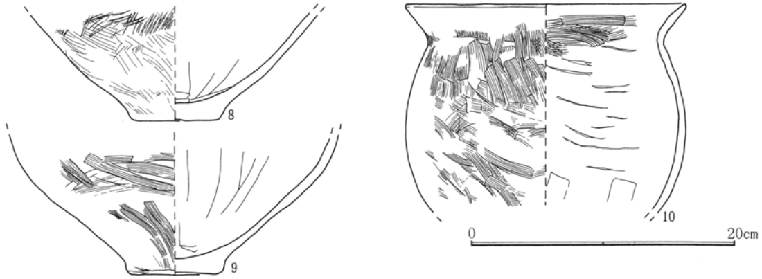
第491図 F-74号住居跡出土遺物(2)
