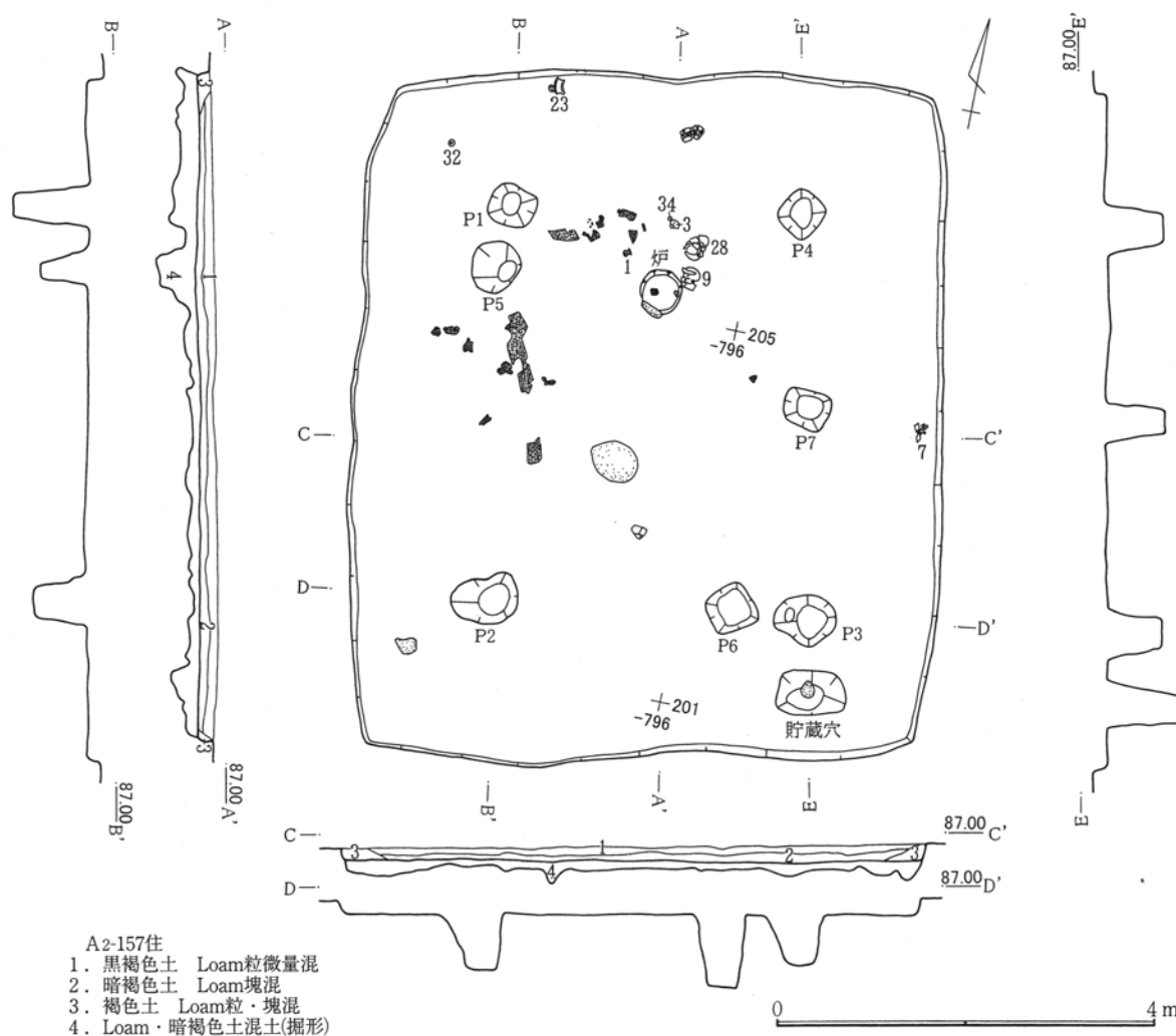
第229図 A2-157号住居跡
