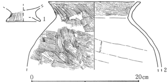
第428図 D3-19号住居跡出土遺物
