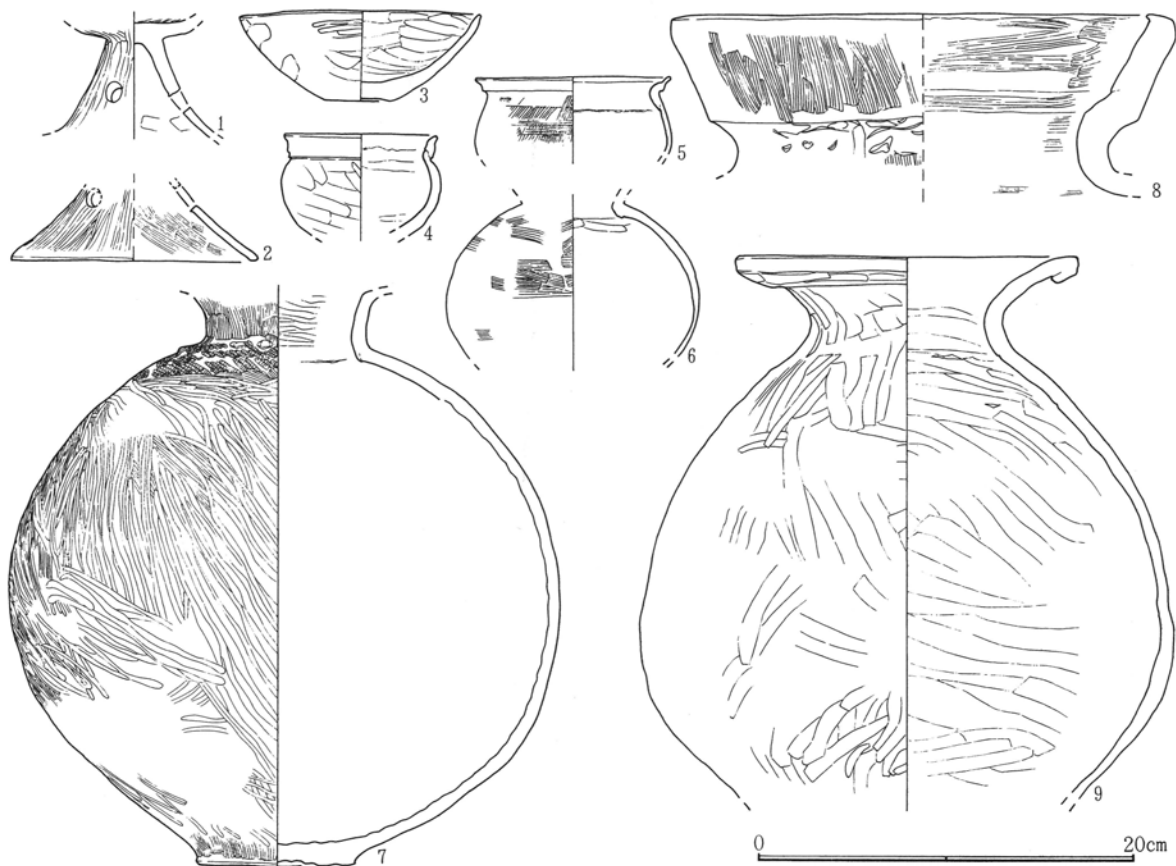
第393図 A 2 -162号住居跡出土遺物(1)
