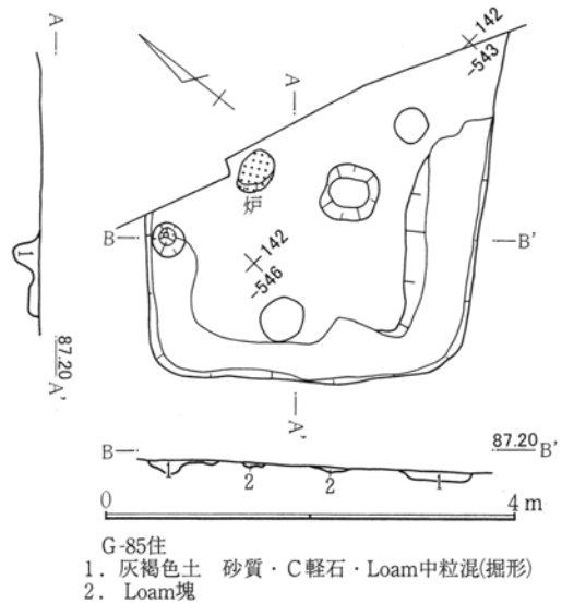
第341図 G-85号住居跡
