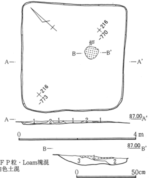
第233図 A2-165号 住居跡
