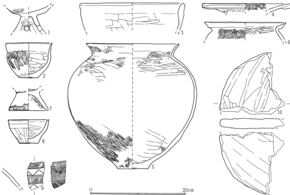
第388図 A 1 -47号住居跡出土遺物
