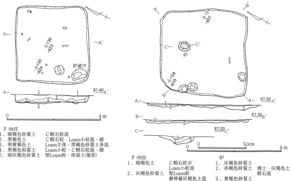
第339図 F-94・95号住居跡
