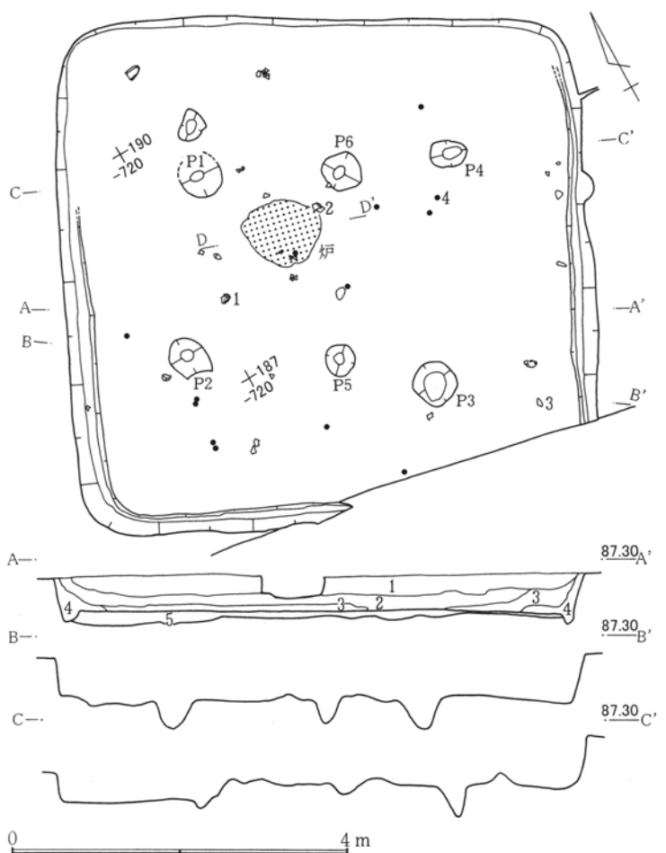
第255図 D3-7号竪穴跡
