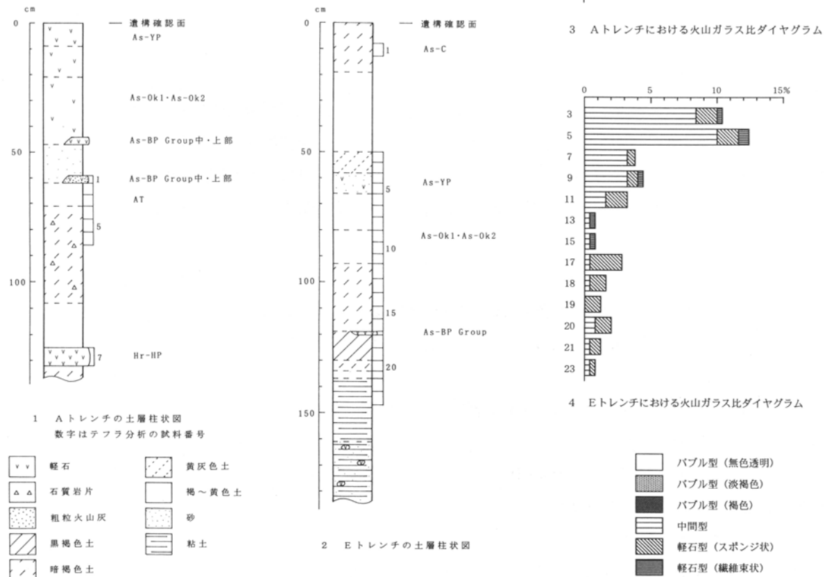
第219図 各試料採取地点の土層柱状図と火山ガラス比ダイアグラム
