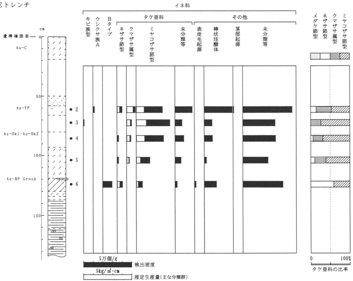
第220図 各トレンチにおける植物珪酸体分析結果
